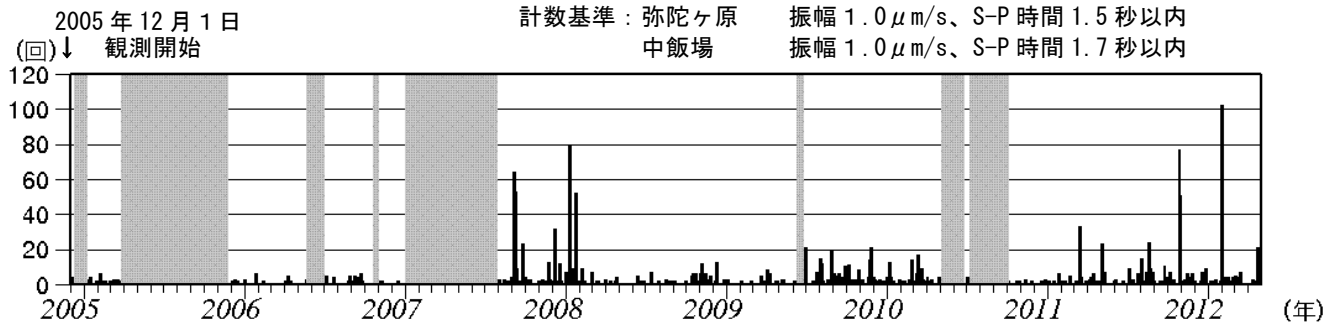
図 3 白山 日別地震回数（2005 年 12 月～2013 年 4 月）
