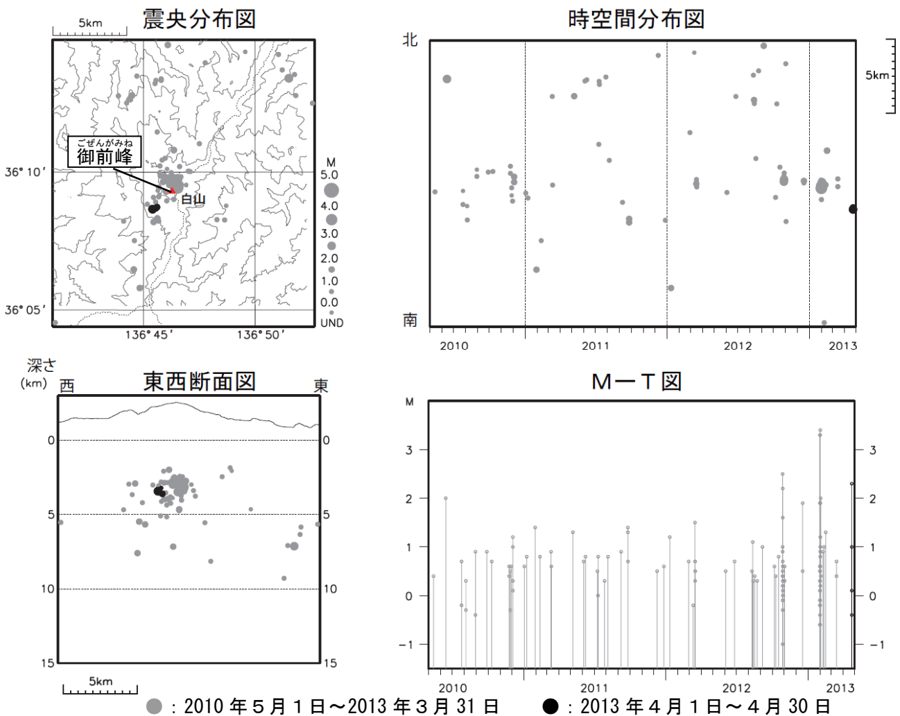
図 4 ※ 白山 広域地震観測網による山体・周辺の地震活動（2010 年 5 月 1 日～2013 年 4 月 30 日）
