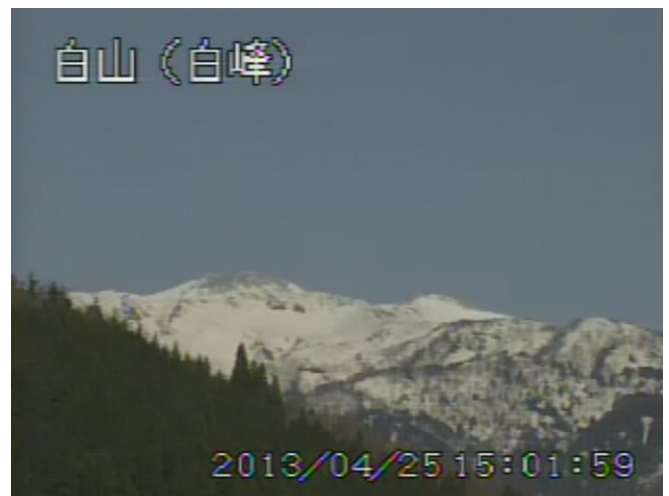
図 2 白山 山頂部の状況 （4 月 25 日 白峰遠望カメラによる）
