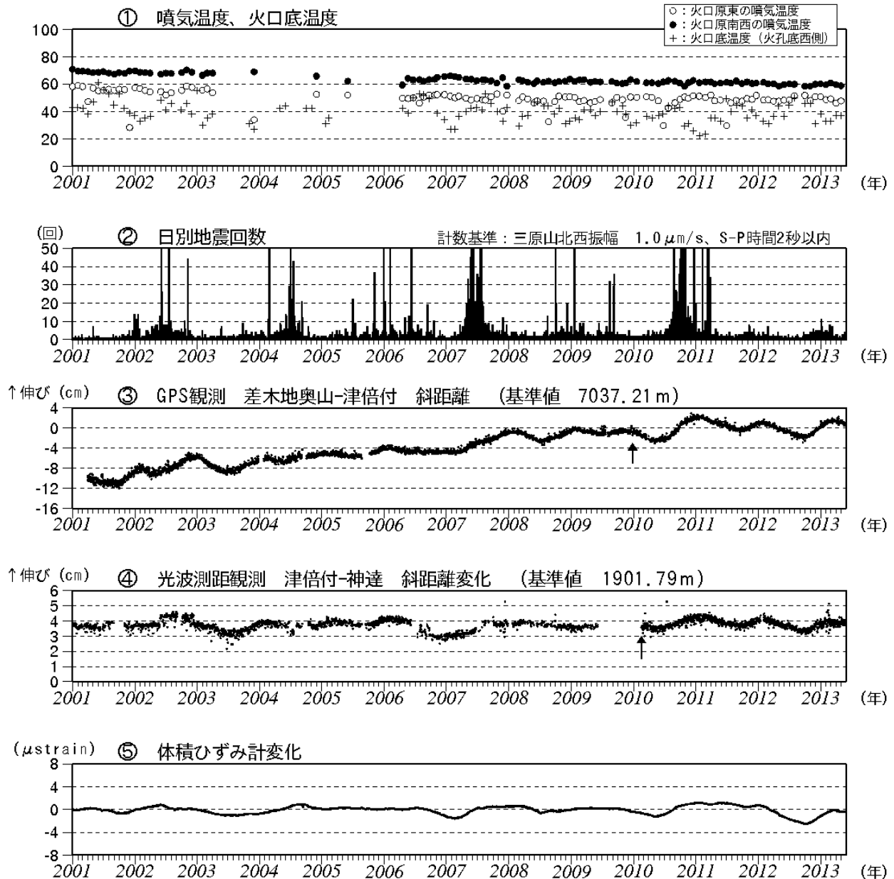
図2 伊豆大島 最近の火山活動経過図（2001年1月～2013年5月）
