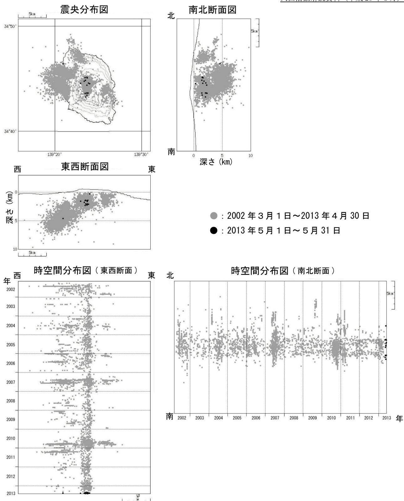
図 7 伊豆大島 震源分布図（2002 年 3 月 1 日～2013 年 5 月 31 日）
