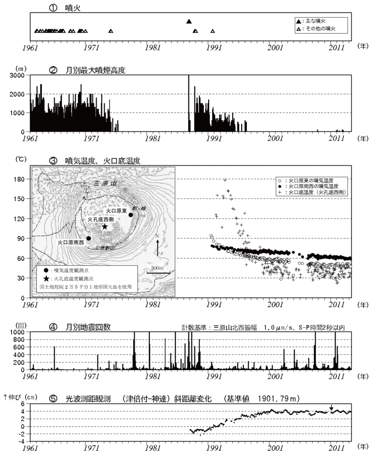
図 1 伊豆大島 長期間の火山活動経過図（1961 年 1 月～2013 年 5 月）
