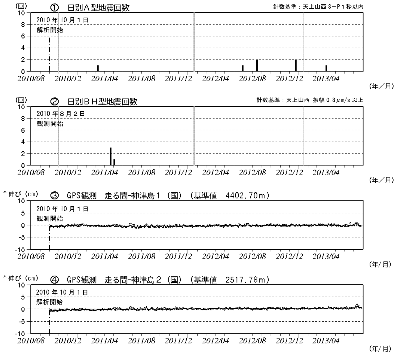
図3 神津島 火山活動経過図(2010年8月2日~2013年7月31日)
