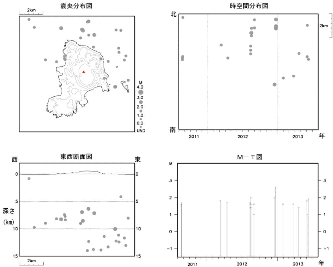
図4 神津島 広域地震観測網による山体・周辺の地震活動（2011 年 8 月 1 日～2013 年 7 月 31 日）
