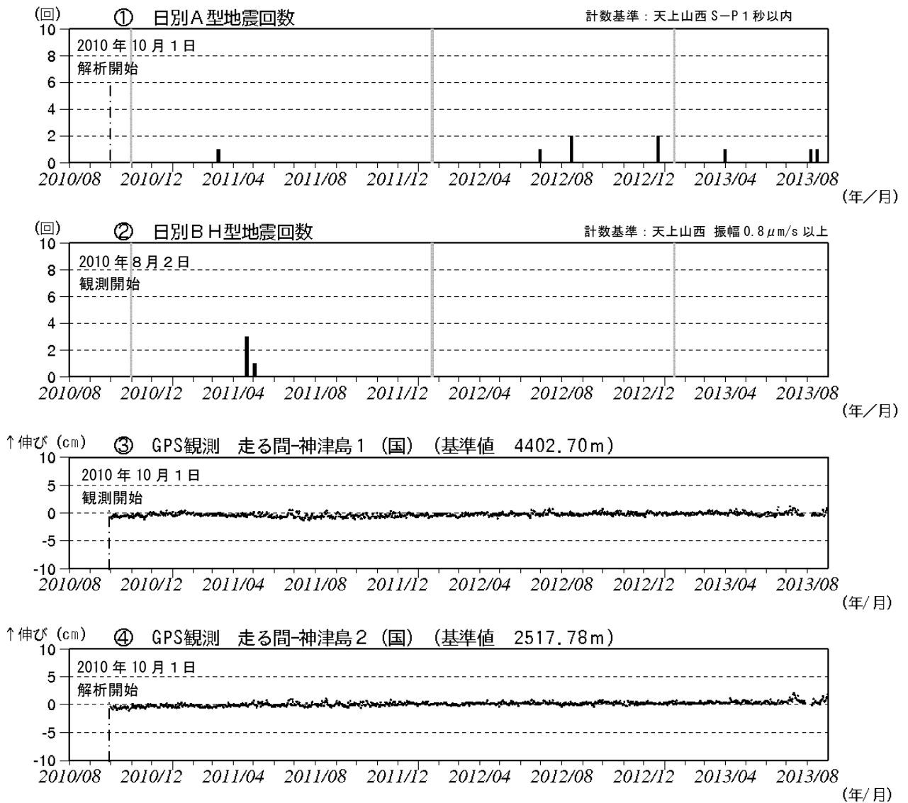
図 3 神津島 火山活動経過図(2010 年 8 月 2 日～2013 年 8 月 31 日)
