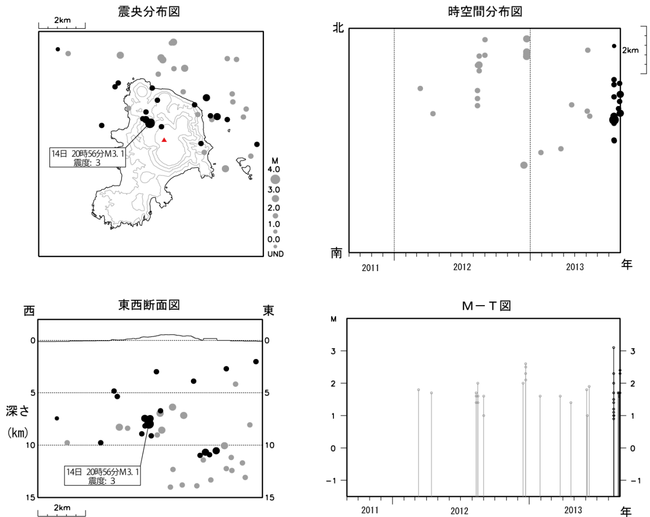
図 4 神津島 広域地震観測網による山体・周辺の地震活動（2011 年 9 月 1 日～2013 年 8 月 31 日）
