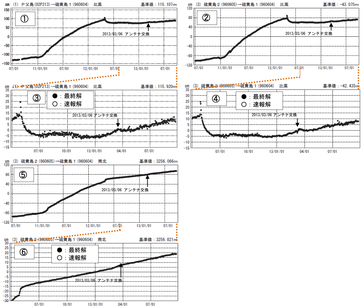
図6 硫黄島 国土地理院による地殻変動観測結果 1) (2010年7月1日～2013年9月22日)
