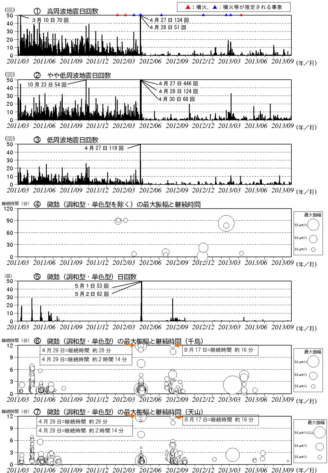
図5 硫黄島 火山活動経過図（2011年3月8日～2013年9月30日）
