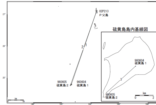
硫黄島周辺 GNSS連続観測基線図
