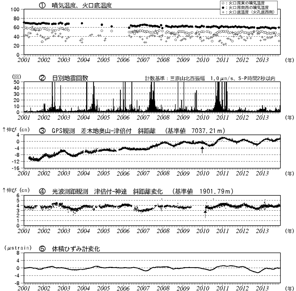
図2 伊豆大島 最近の火山活動経過図（2001年1月～2013年11月）
