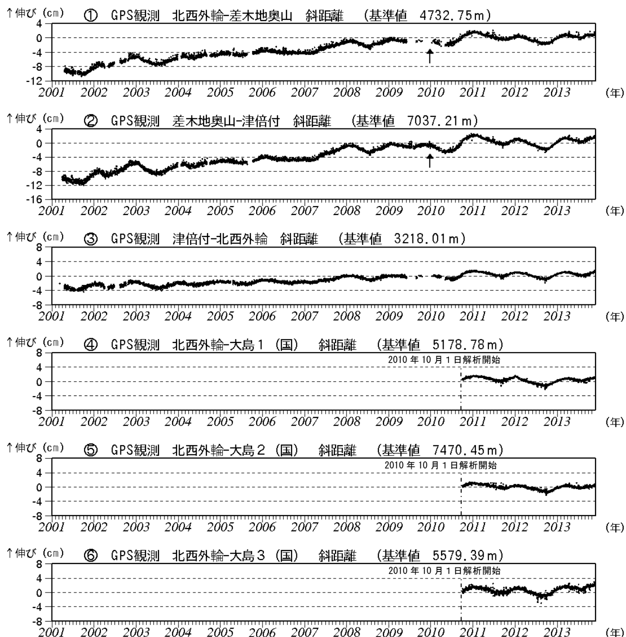
図3 伊豆大島 GPS連続観測による基線長変化(2001年1月～2013年11月) (国): 国土地理院 2010年10月以降のデータについては、電離層の影響を補正する等、解析方法を改良しています。 ①～⑥は図8のGPS基線①～⑥に対応しています。 グラフの空白部分は欠測。 ①②の矢印は差木地奥山支柱工事を実施。
