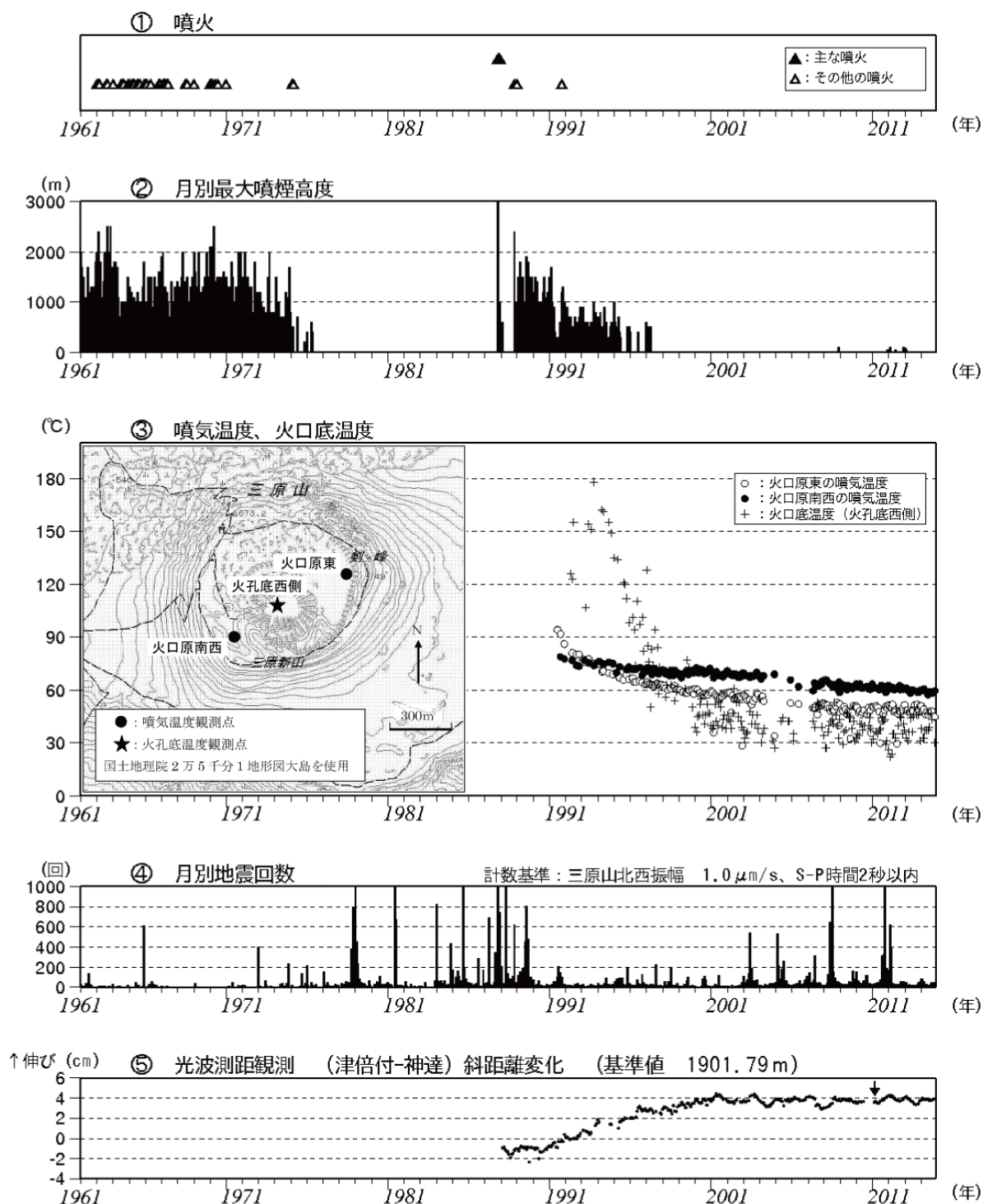
図1 伊豆大島 長期間の火山活動経過図（1961年1月～2013年11月）
