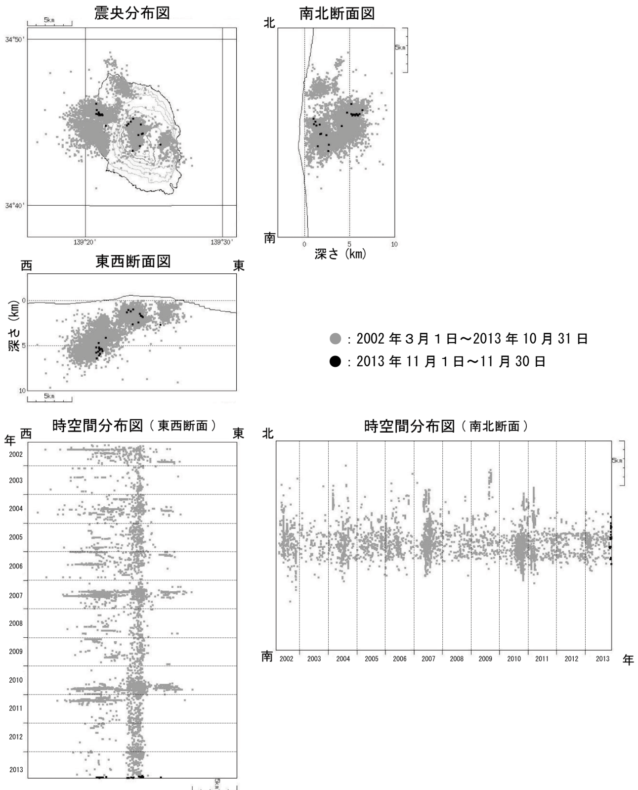
図 7 伊豆大島 震源分布図（2002 年 3 月 1 日～2013 年 11 月 30 日）
