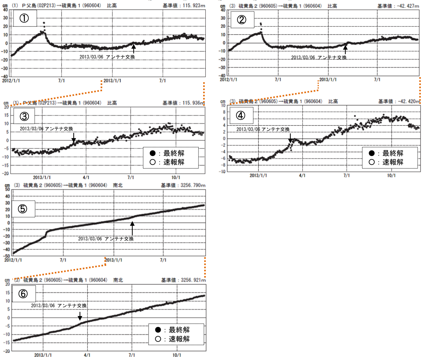
図 6 硫黄島 国土地理院による地殻変動観測結果 1) (2012 年 1 月 1 日～2013 年 11 月 25 日)
