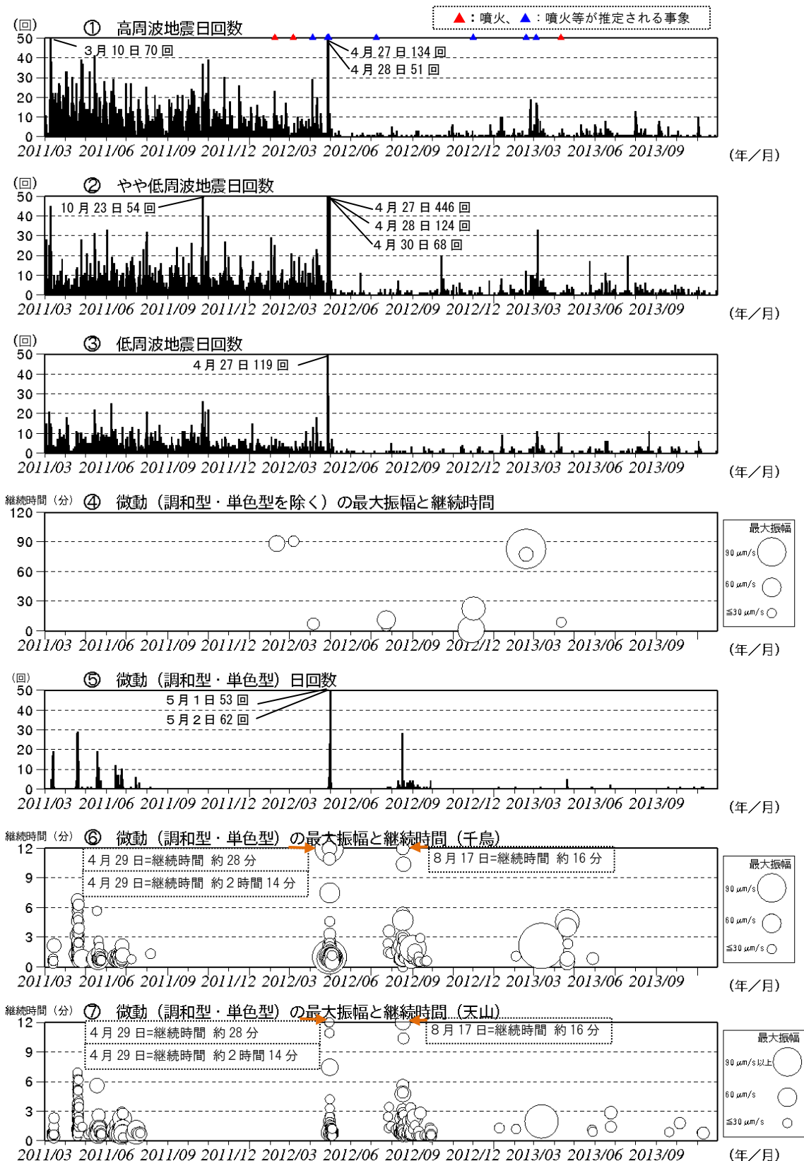
図5 硫黄島 火山活動経過図（2011年3月8日～2013年11月30日）
