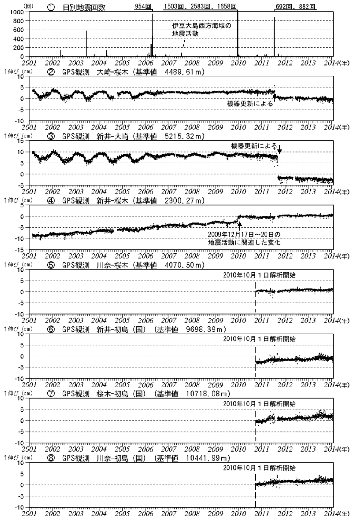
図3 伊豆東部火山群 最近の火山活動経過図（2001年1月～2014年1月）
