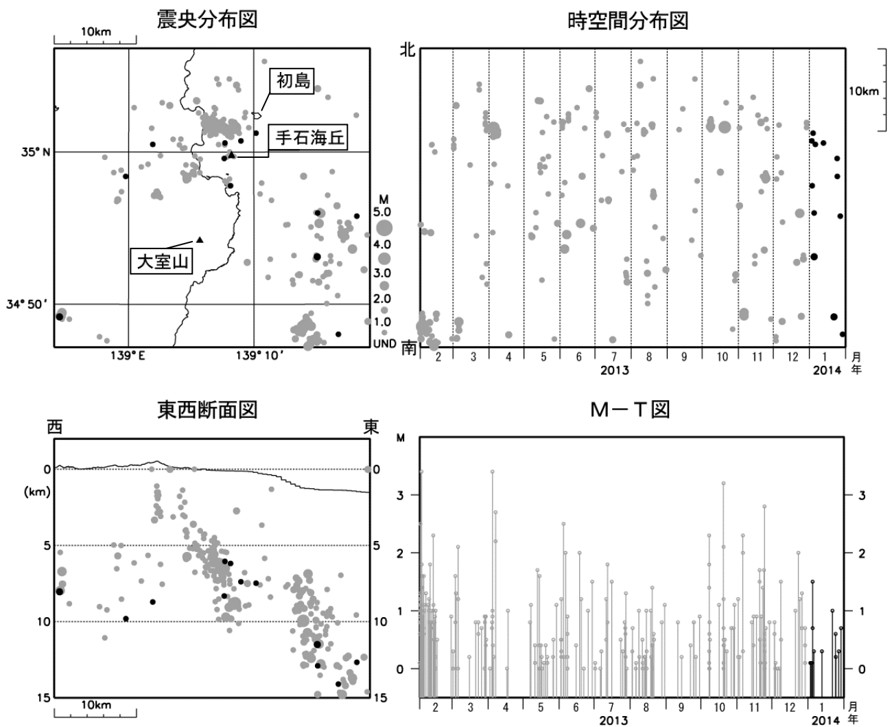
図 2 伊豆東部火山群 広域地震観測網による震源分布図（2013 年 2 月 1 日～2014 年 1 月 31 日）
