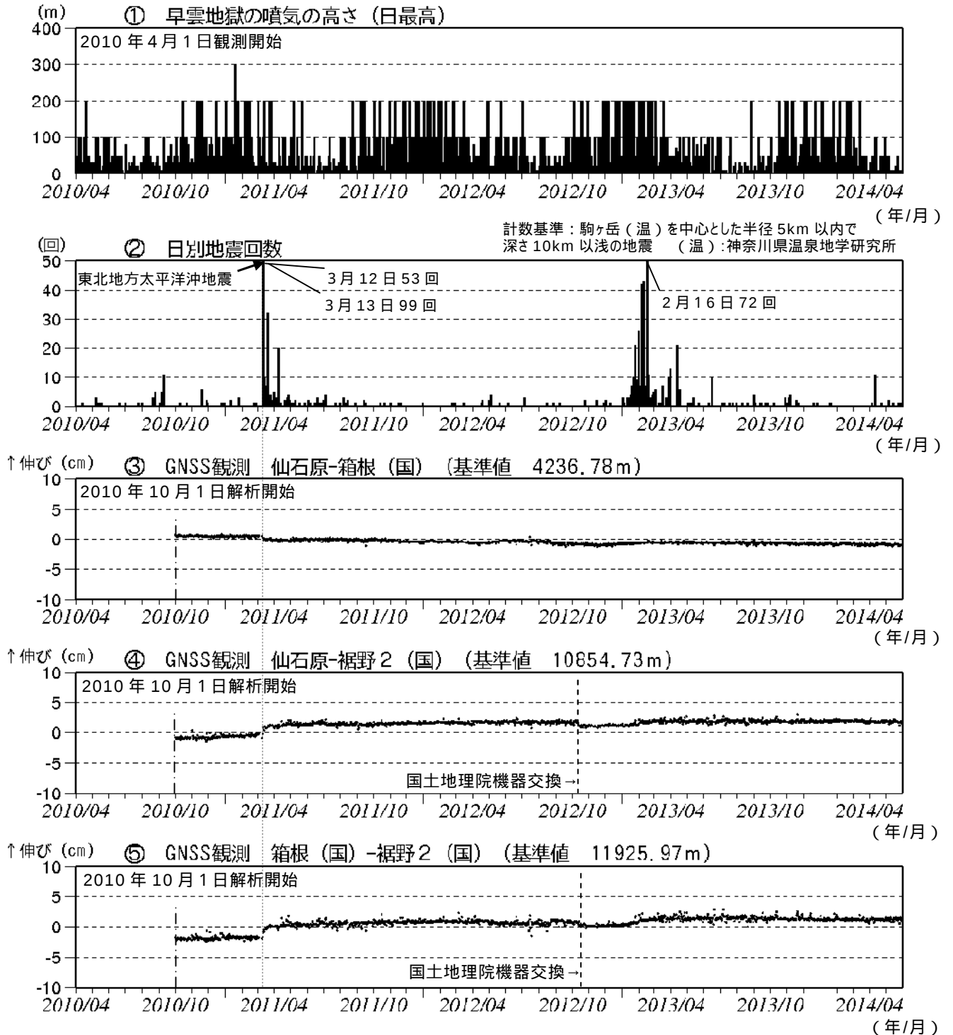
図 4 箱根山 火山活動経過図（2010 年 4 月 1 日～2014 年 5 月 31 日）
