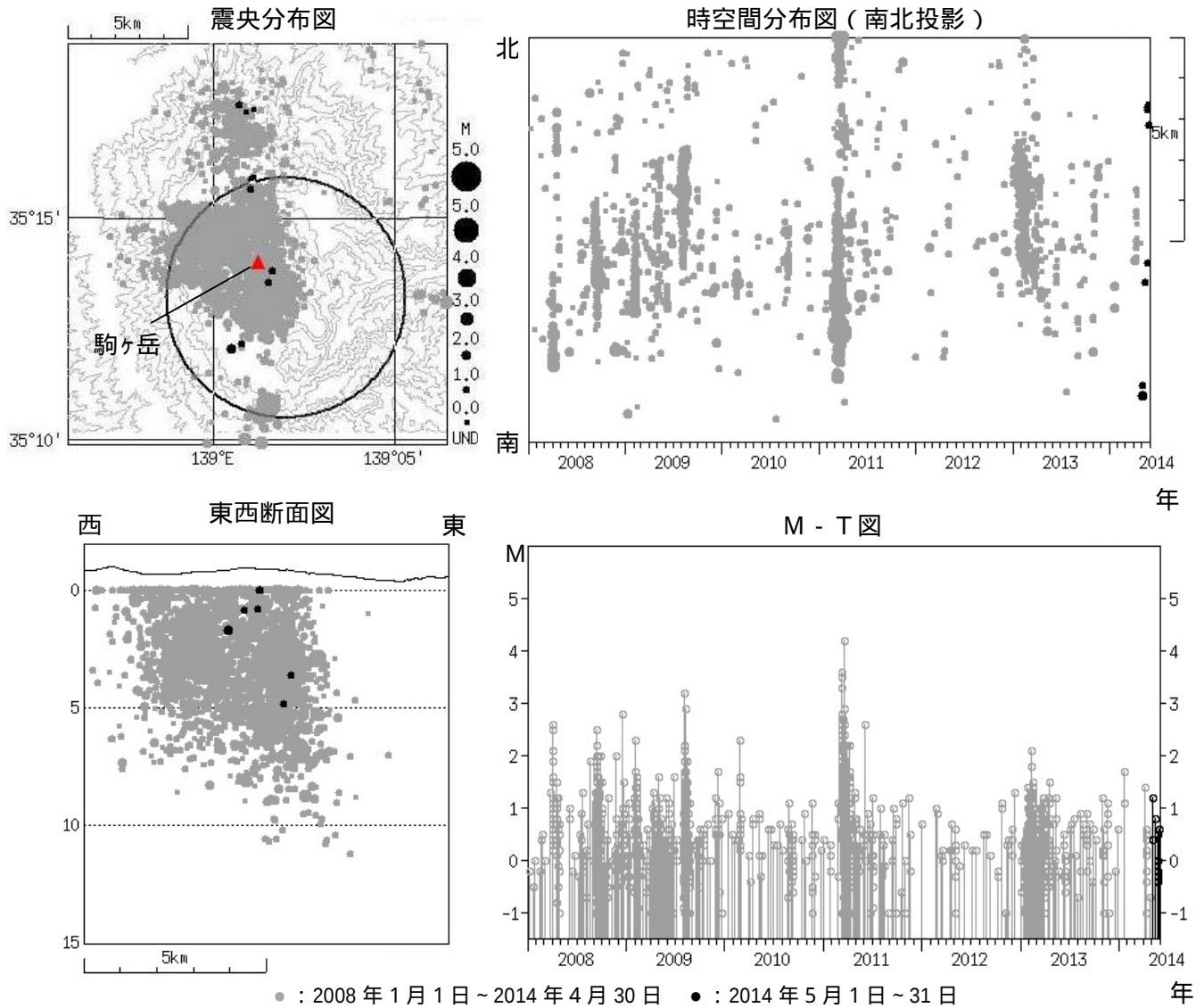
図 5 箱根山 広域地震観測網による山体周辺の震源分布図（2008 年 1 月 1 日 ~ 2014 年 5 月 31 日） M（マグニチュード）は地震の規模を表します。 図中の震源要素は一部暫定値が含まれており、後日変更することがあります。 震源分布図の円は、駒ヶ岳観測点（温）を中心とした半径 5 km の範囲を示しています。
