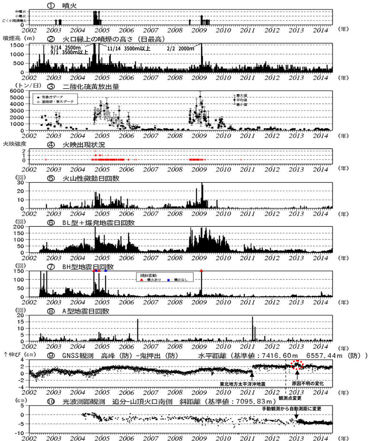
図3 浅間山 火山活動経過図（2002 年 1 月 1 日～2014 年 6 月 30 日）
