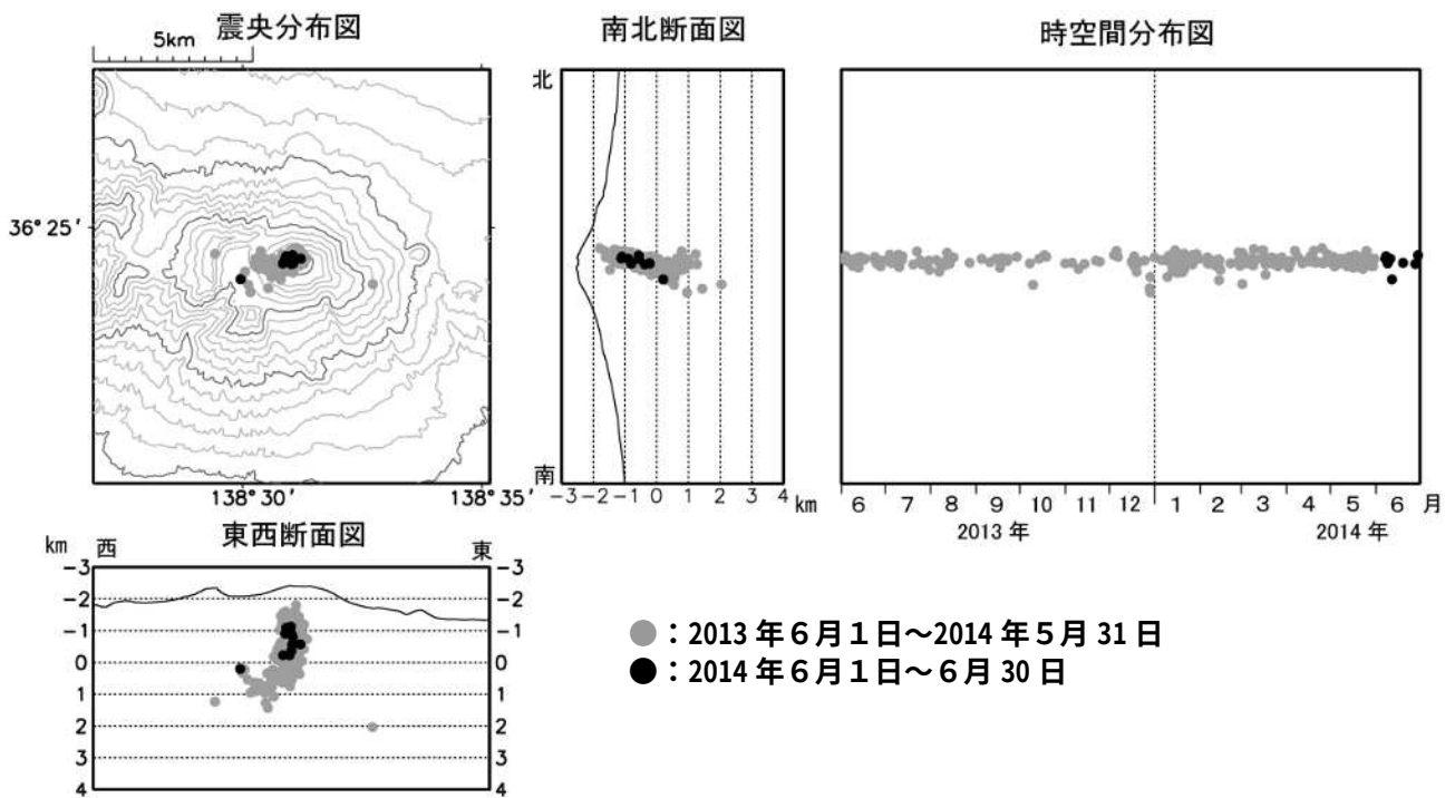
図 4 浅間山 震源分布図（2013 年 6 月 1 日～2014 年 6 月 30 日）
