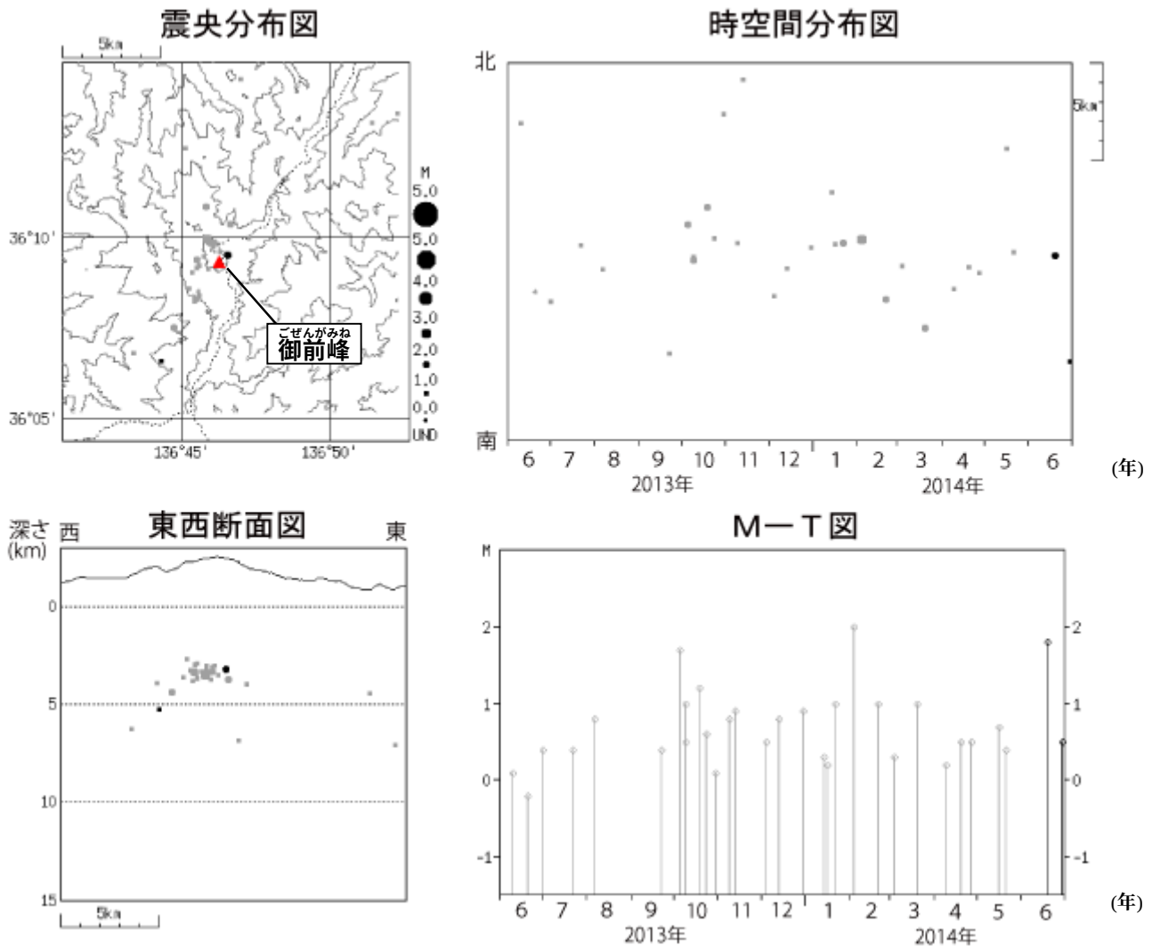
図4 白山 広域地震観測網による山体・周辺の地震活動 (2013 年 6 月 1 日～2014 年 6 月 30 日)
