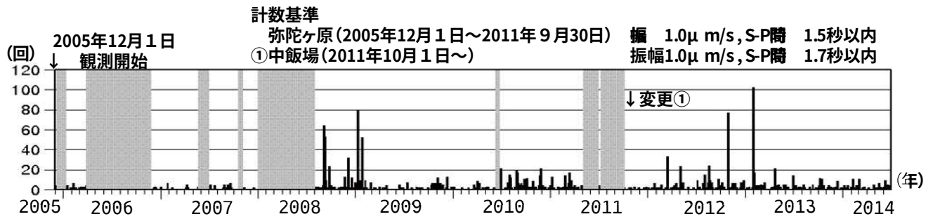
図3 白山 日別地震回数 (2005 年 12 月 1 日～2014 年 6 月 30 日)
