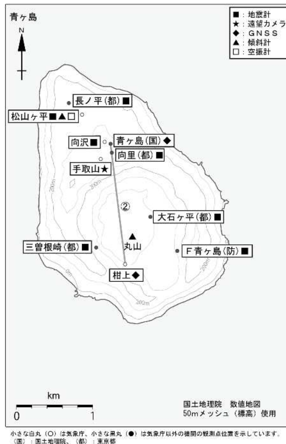
図 3 青ヶ島 観測点配置図
