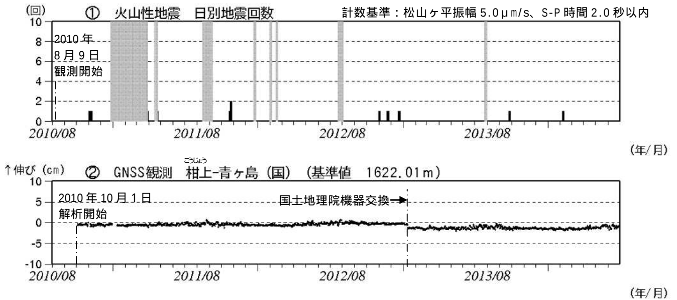
図 2 青ヶ島 火山活動経過図（2010 年 8 月 9 日～2014 年 6 月 30 日）
