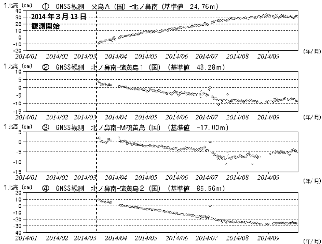
図 7 硫黄島 GNSS 2) 観測結果（2014 年 1 月～9 月）（国）：国土地理院
