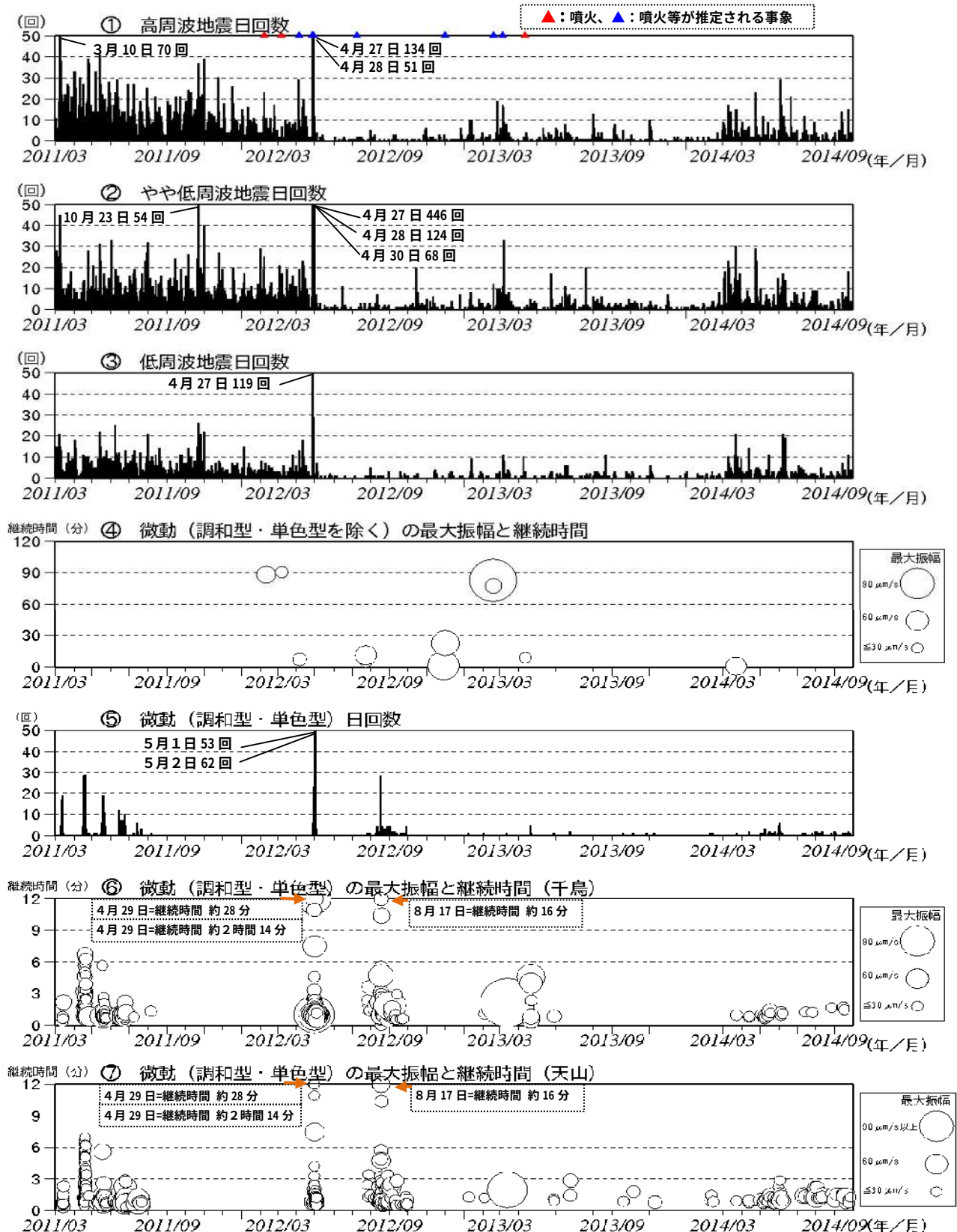
図5 硫黄島 火山活動経過図（2011年3月8日～2014年9月30日）
