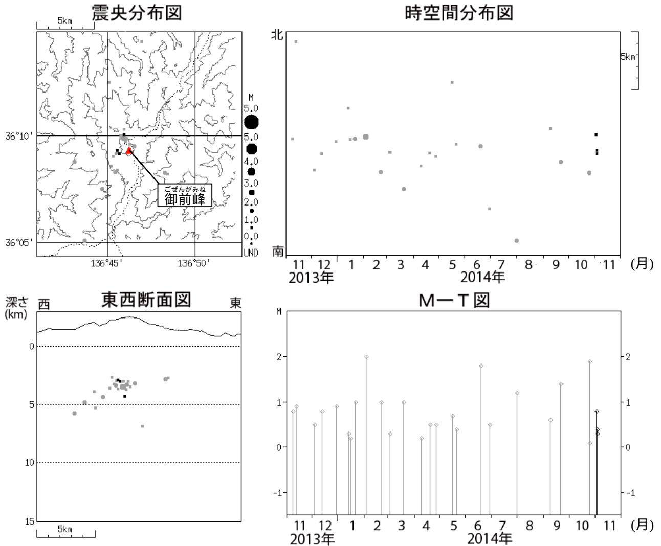
図4 白山 広域地震観測網による山体・周辺の地震活動（2013年11月1日～2014年11月30日）
