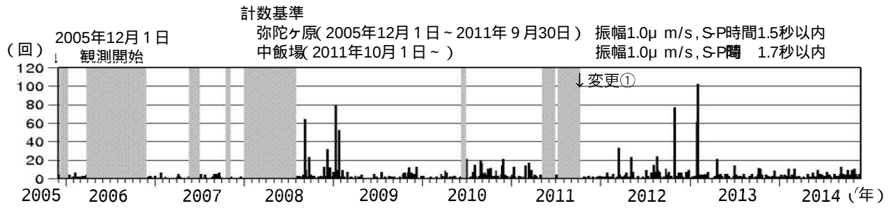
図3 白山 日別地震回数（2005年12月1日～2014年11月30日）
