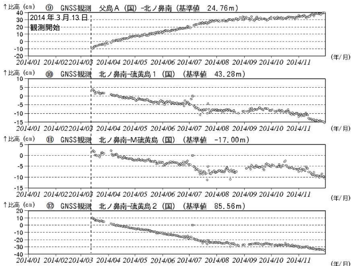
図7 硫黄島 GNSS 1) 観測結果(2014年1月~11月) (国): 国土地理院
