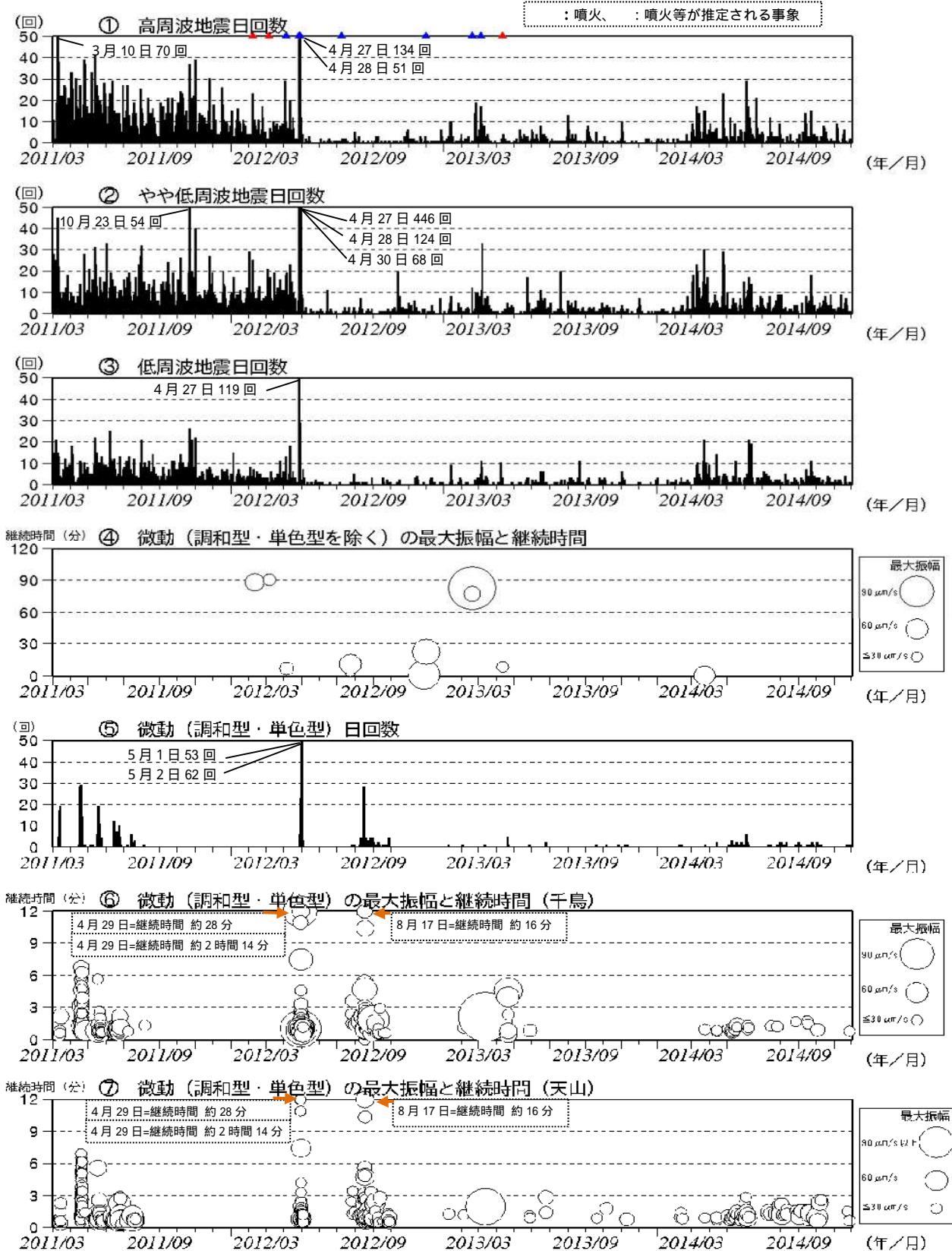
図5 硫黄島 火山活動経過図(2011年3月8日~2014年11月30日)
