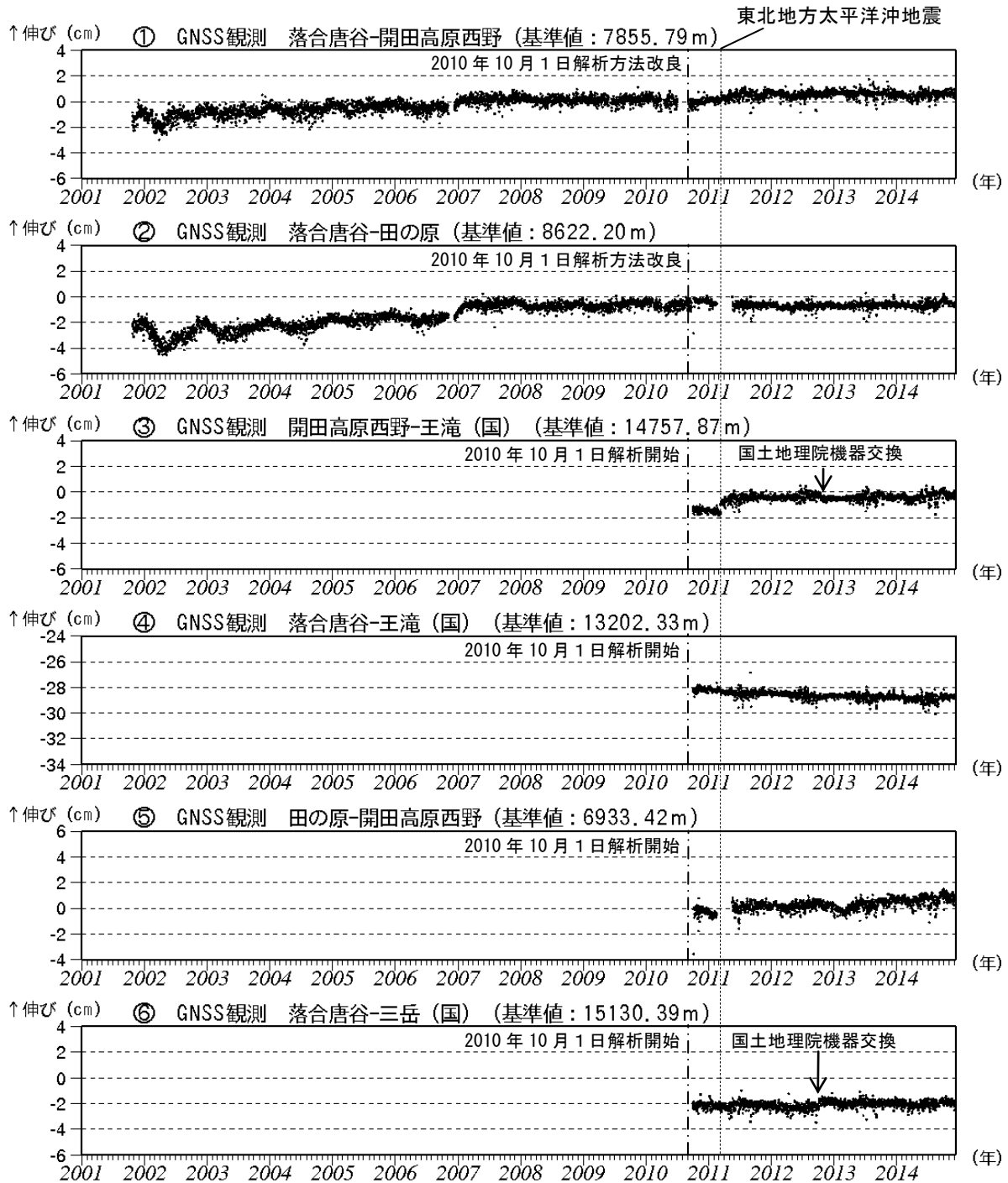
図3 御嶽山 GNSS連続観測による基線長の長期変化 (2001年1月1日～2014年12月10日)
