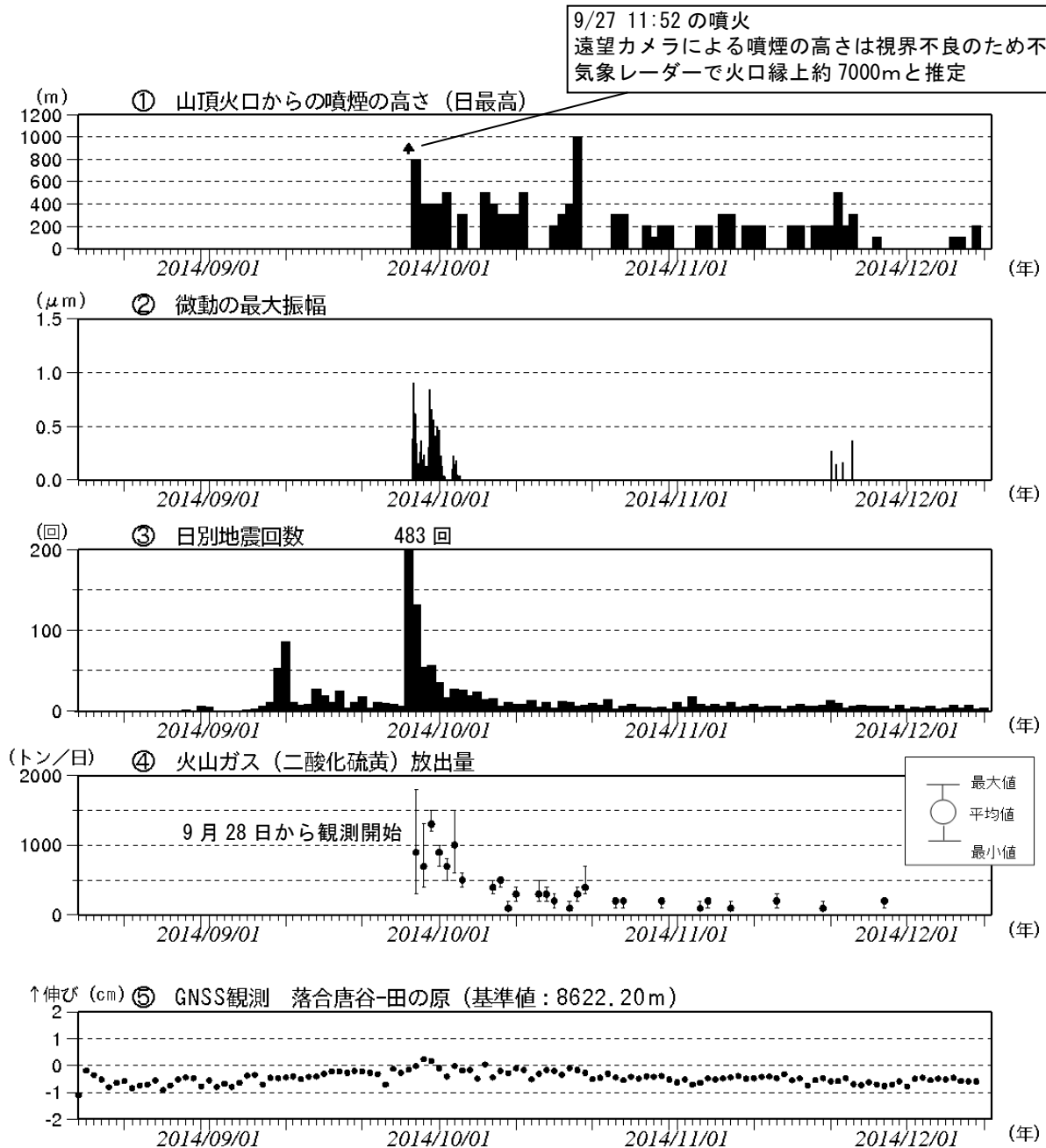
図 2 御嶽山 日別活動状況（2014 年 8 月 15 日～12 月 11 日（速報値含む））
