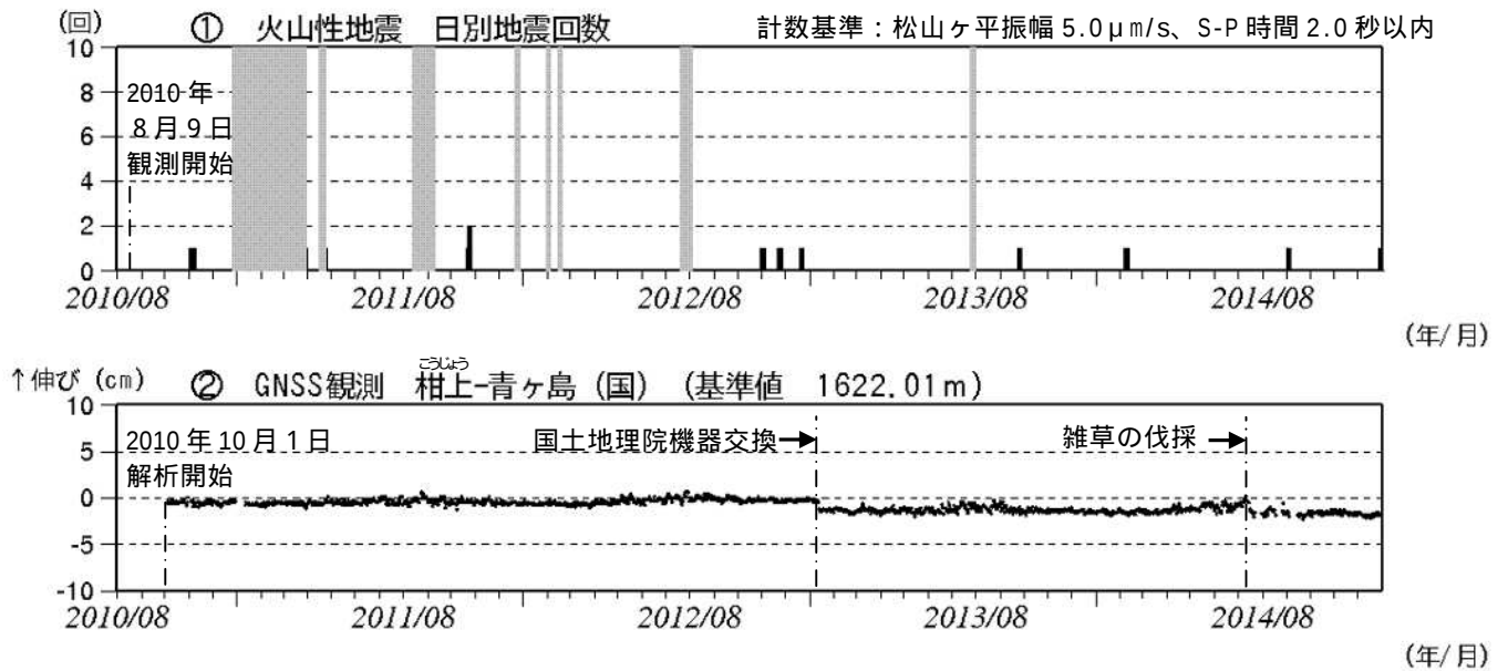
図2 青ヶ島 火山活動経過図（2010年8月9日～2014年12月31日）
