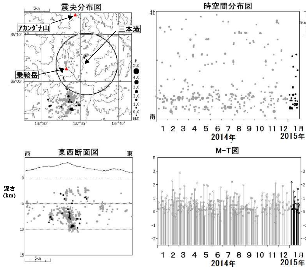
図3 乗鞍岳 広域地震観測網による山体・周辺の地震活動(2014 年 1 月 1 日～2015 年 1 月 31 日)
