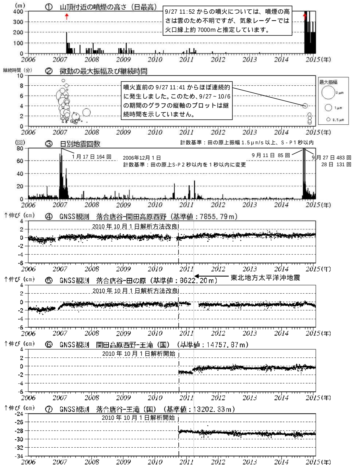
図 4 御嶽山 長期間の火山活動経過図（2006 年 1 月 1 日～2015 年 1 月 31 日）
