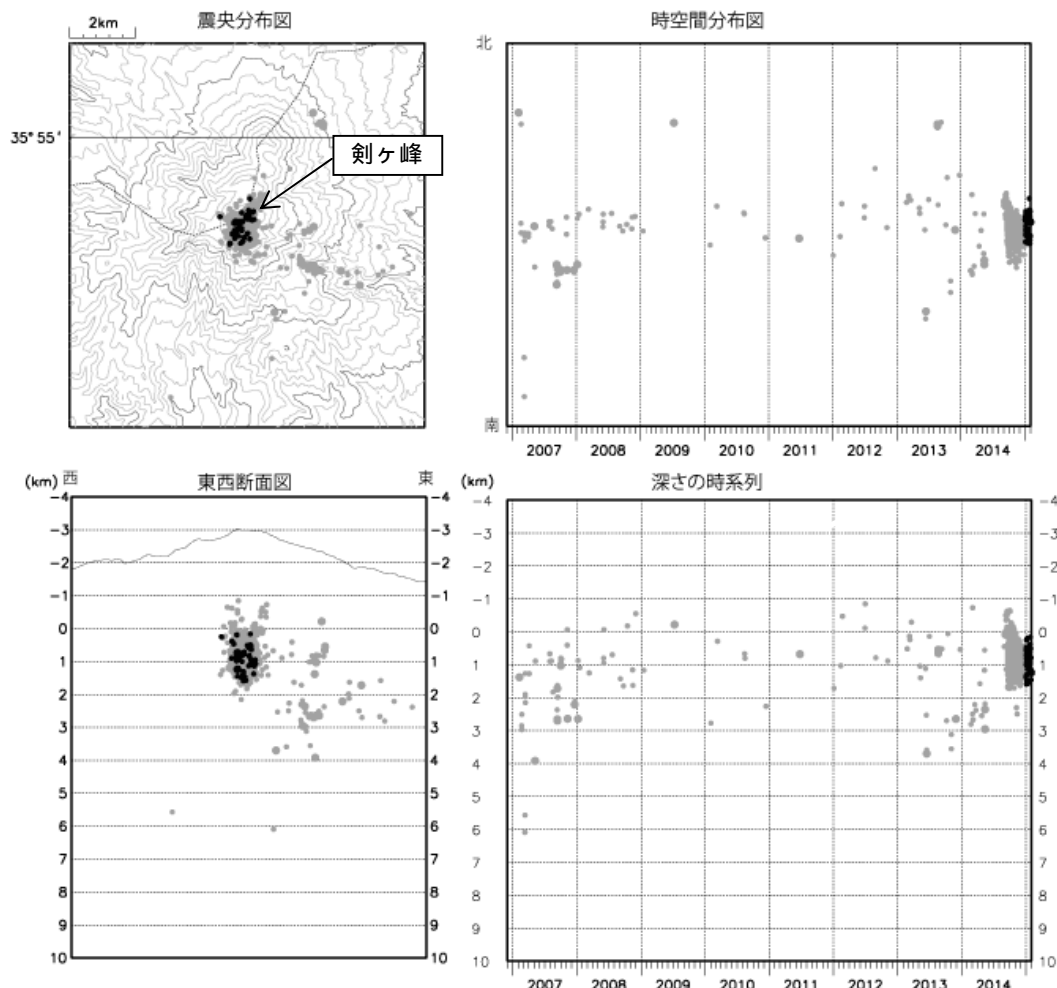
図 2 御嶽山 震源分布図（2006 年 12 月 1 日～2015 年 1 月 31 日）
