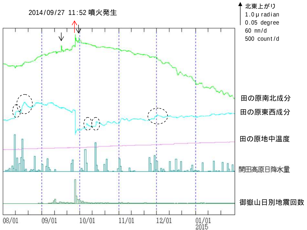
図5 御嶽山 田の原観測点（剣ヶ峰山頂の南東約3 km）の傾斜変動 （2014年8月1日～2015年1月31日）
