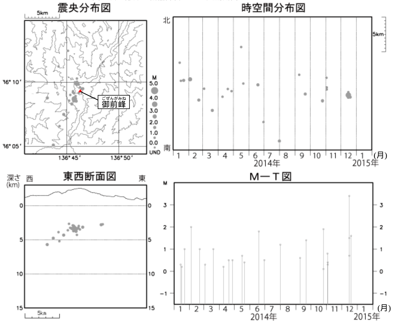
図 4 白山 広域地震観測網による山体・周辺の地震活動（2014 年 1 月 1 日～2015 年 1 月 31 日）
