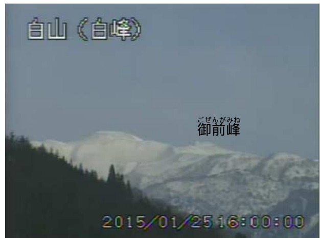
図 2 白山 山頂部の状況 （1 月 25 日 白峰遠望カメラによる）
