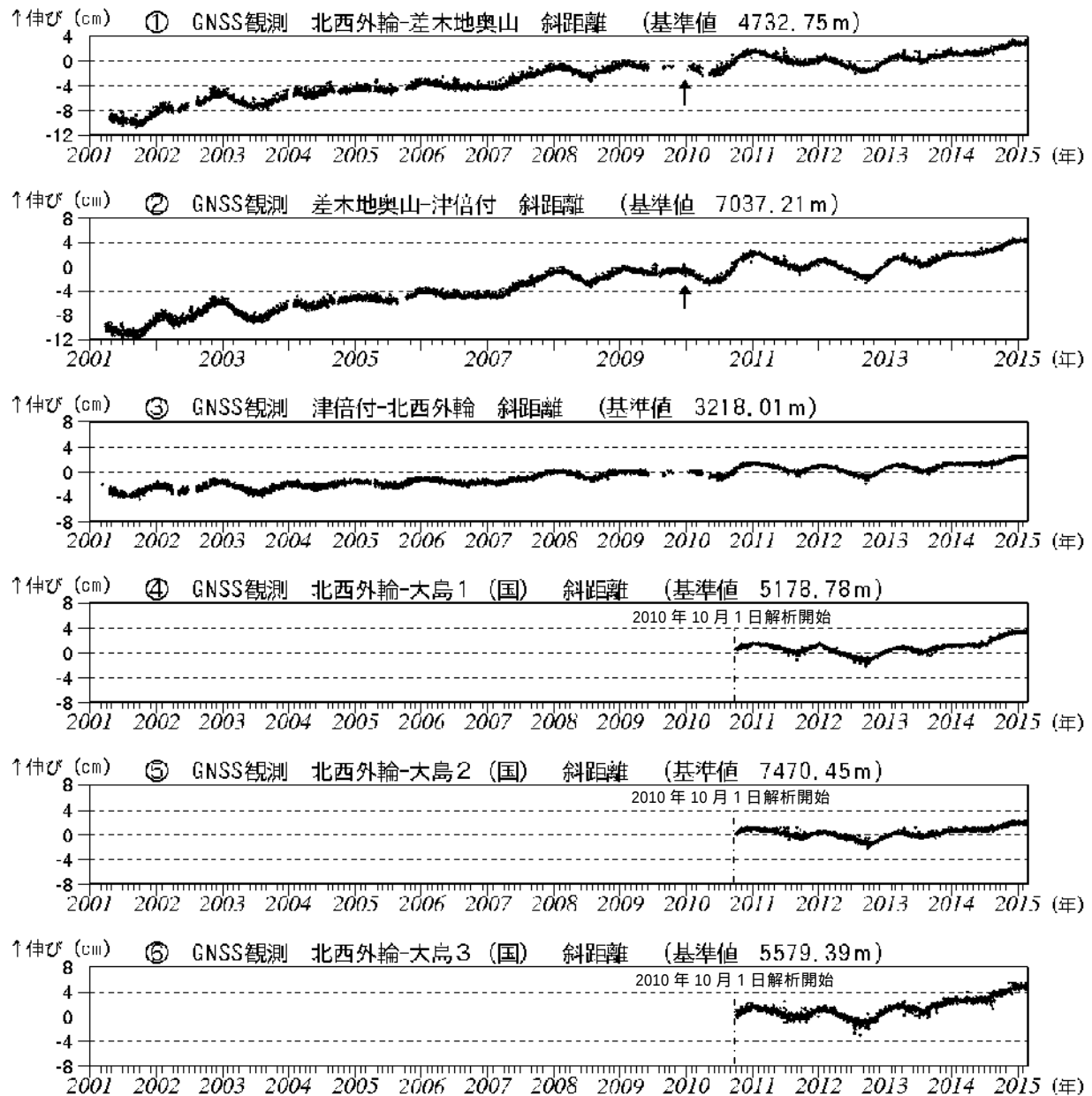
図3 伊豆大島 GNSS連続観測による基線長変化(2001年1月~2015年2月28日)(国): 国土地理院
