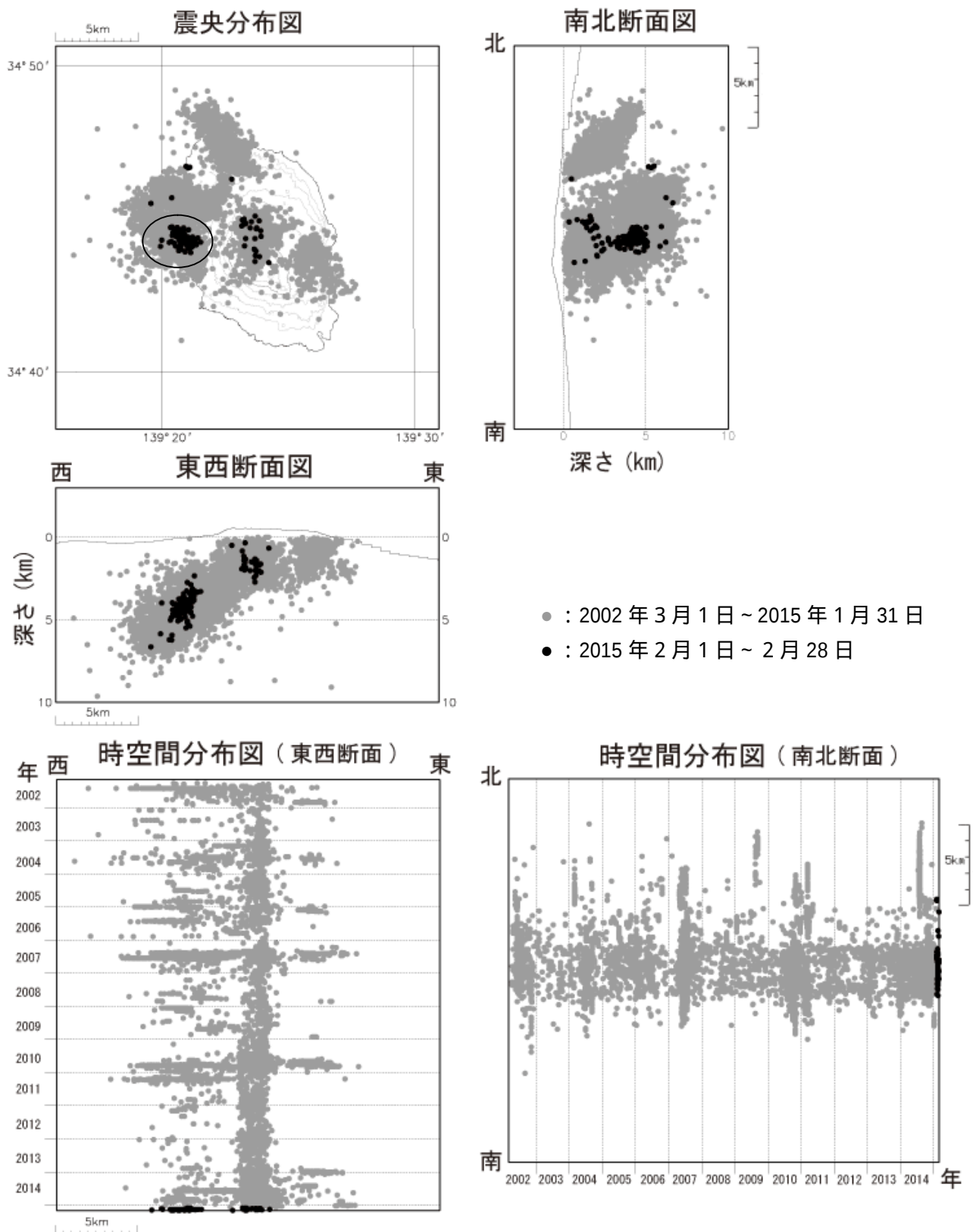
図 4 伊豆大島 震源分布図（2002 年 3 月 1 日～2015 年 2 月 28 日）
