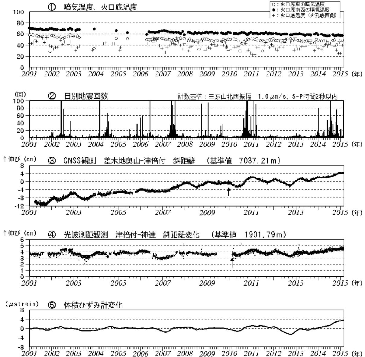
図2 伊豆大島 最近の火山活動経過図（2001年1月～2015年2月28日）
