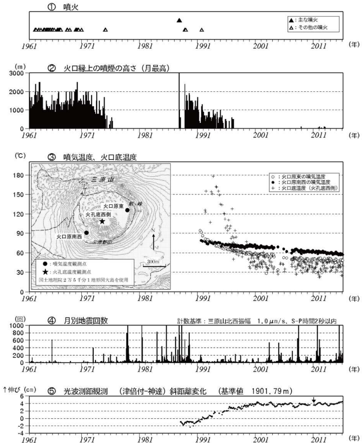
図 1 伊豆大島 長期間の火山活動経過図（1961 年 1 月～2015 年 2 月 28 日）
