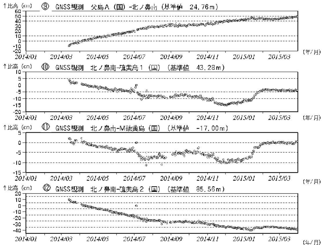
図7 硫黄島 GNSS 2) 観測結果（2014 年 1 月～2015 年 3 月）（国）：国土地理院
