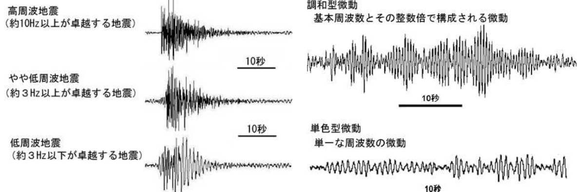
図 4 硫黄島でみられる主な火山性地震、微動（調和型、単色型）の特徴と波形例
