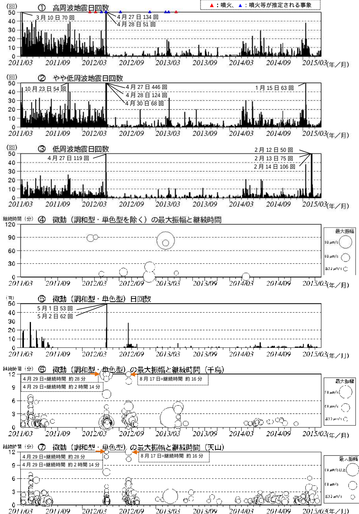
図5 硫黄島 火山活動経過図（2011年3月8日～2015年3月31日）
