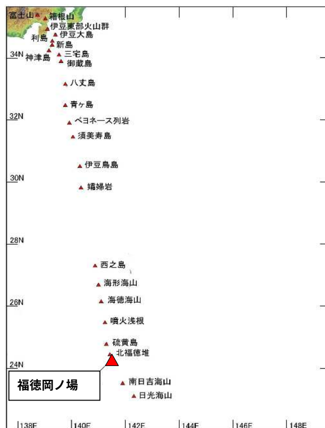
図 1 福徳岡ノ場 伊豆・小笠原諸島の活火山分布と福徳岡ノ場 地図は、日本活火山総覧（第 4 版）から引用。
