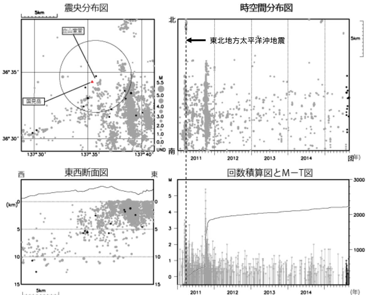
図 1 弥陀ヶ原 広域地震観測網による山体・周辺の地震活動（2011 年 1 月 1 日～2015 年 8 月 31 日）
