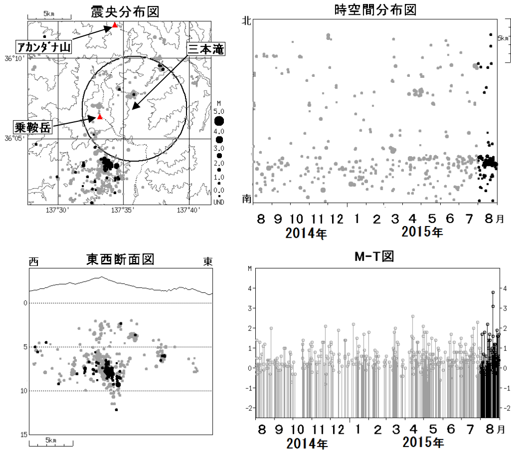
図 3 乗鞍岳 広域地震観測網による山体・周辺の地震活動(2014 年 8 月 1 日～2015 年 8 月 31 日)
