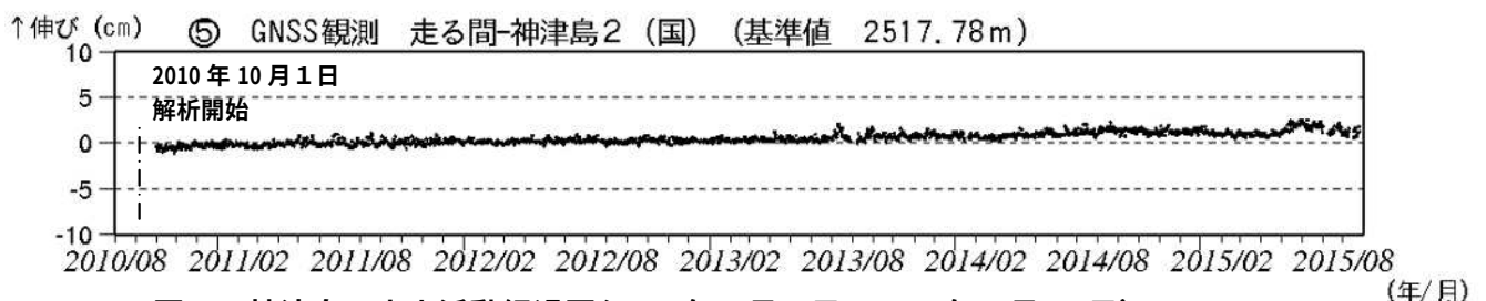
図3 神津島 火山活動経過図(2010年8月2日～2015年8月31日)
