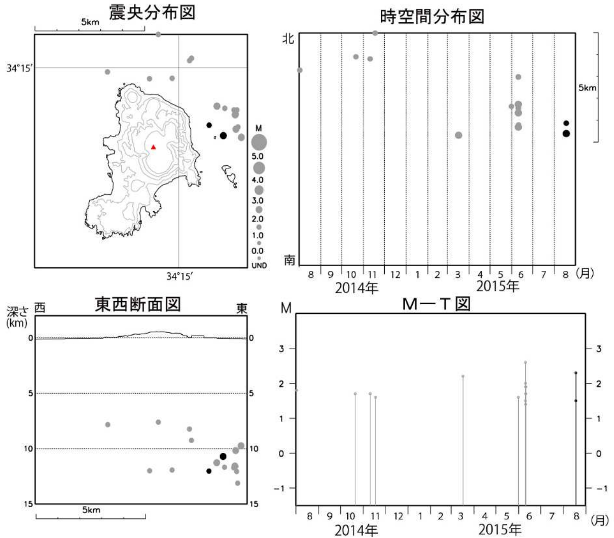
図4 神津島 広域地震観測網による山体・周辺の地震活動（2014 年 8 月 1 日～2015 年 8 月 31 日）
