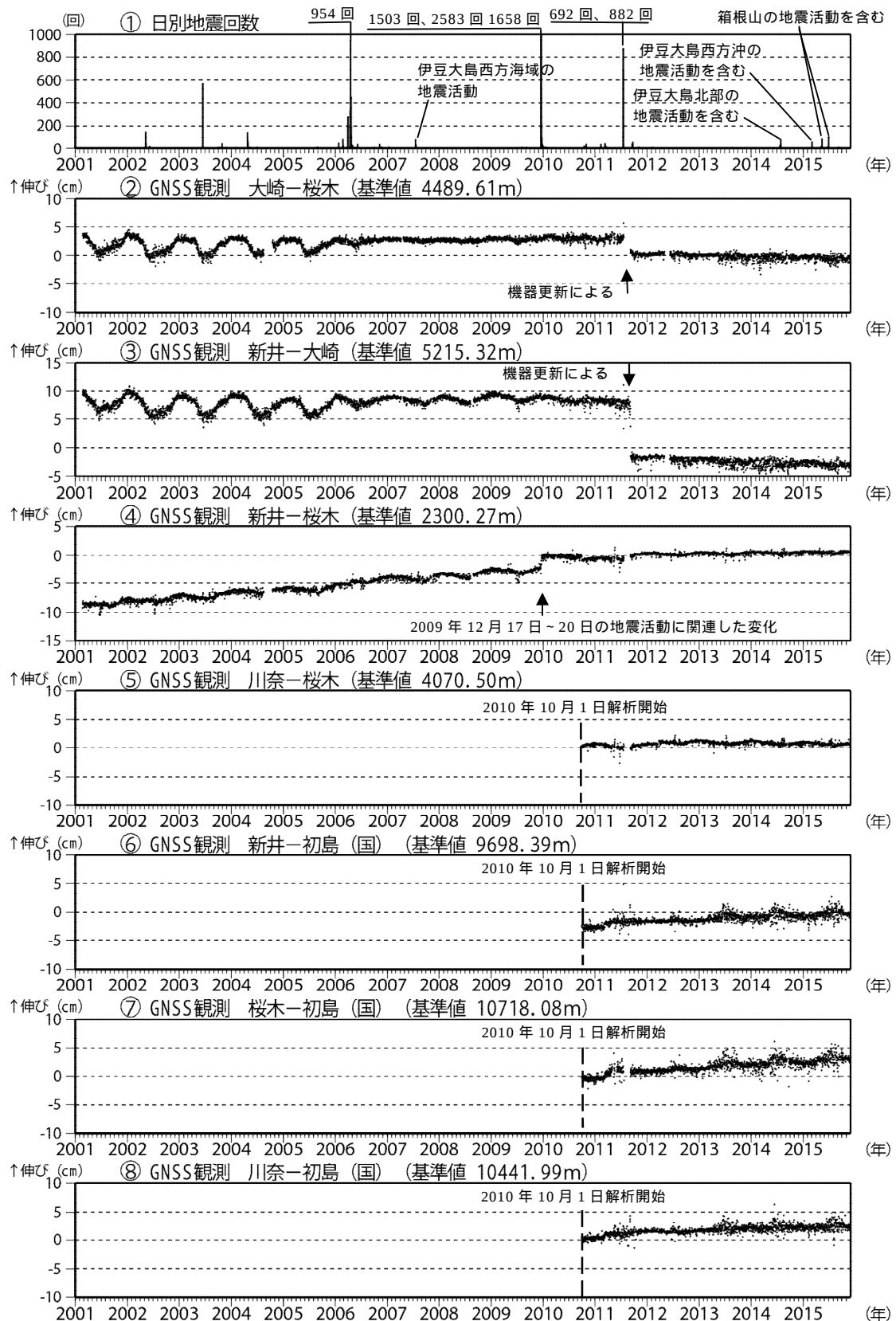
図3 伊豆東部火山群 火山活動経過図（2001年1月1日～2015年11月30日）
