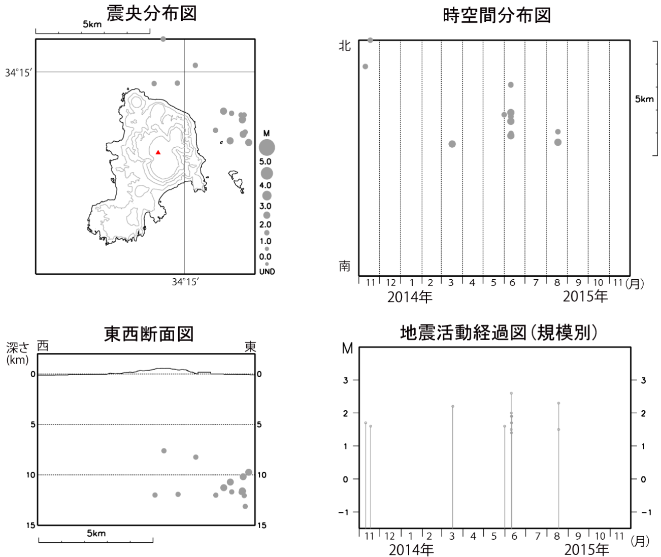
図 4 神津島 広域地震観測網による山体・周辺の地震活動（2014 年 11 月 1 日～2015 年 11 月 30 日）
