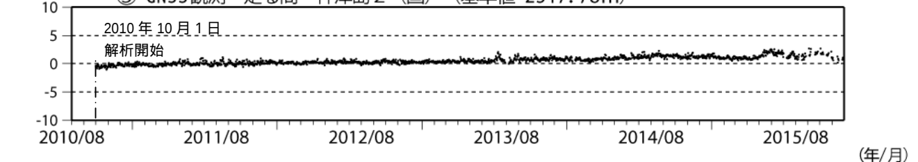
図 3 神津島 火山活動経過図(2010 年 8 月 2 日～2015 年 11 月 30 日)
