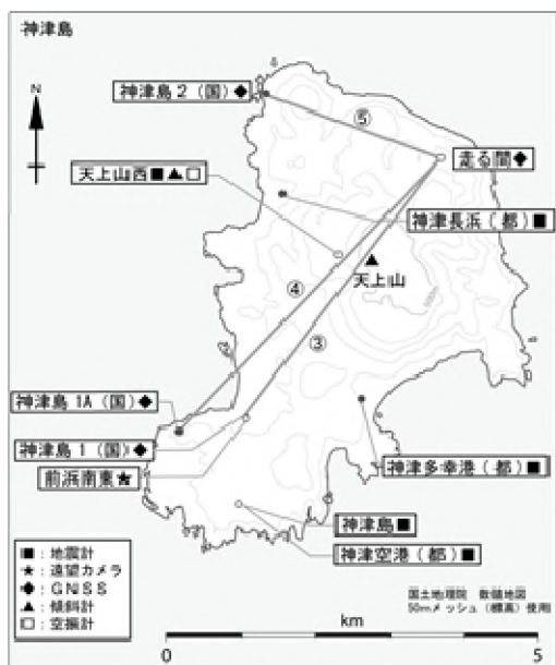
図1 神津島 観測点配置図
