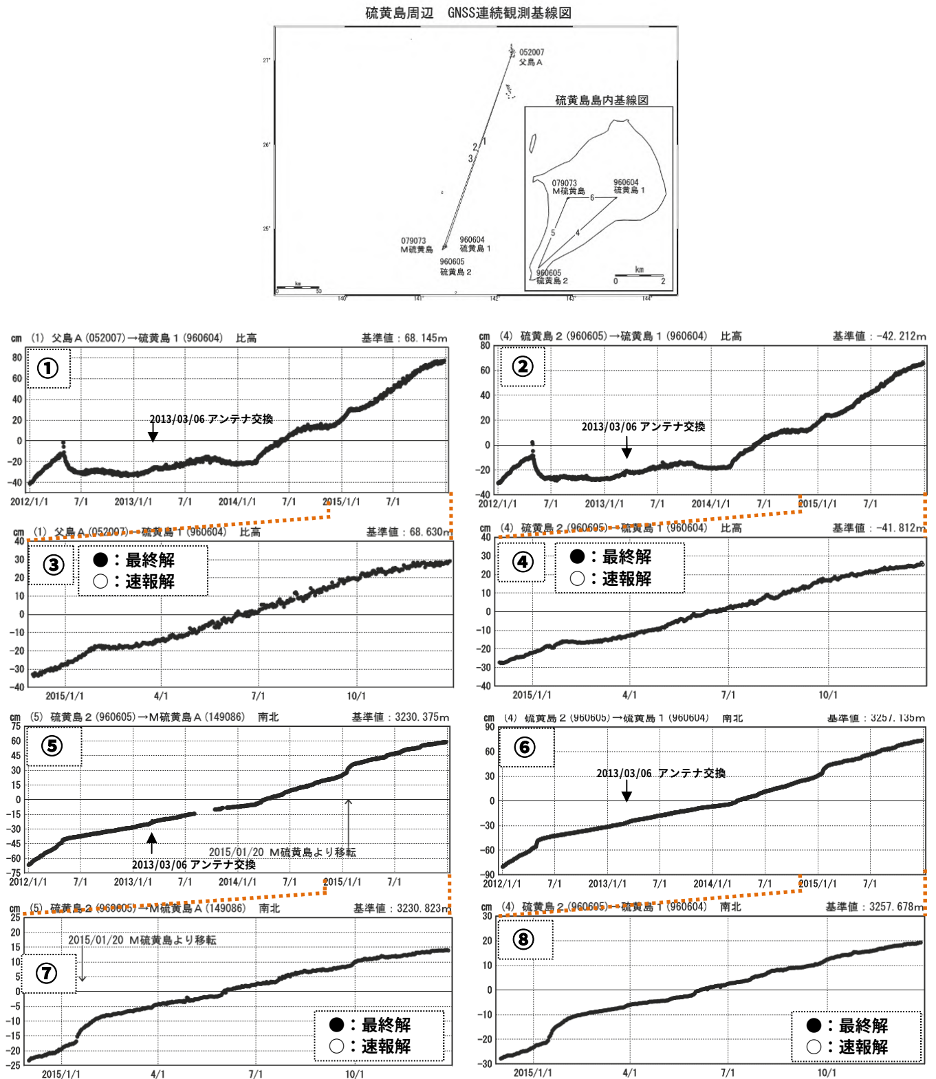
図 8 硫黄島 国土地理院による地殻変動観測結果 2)
