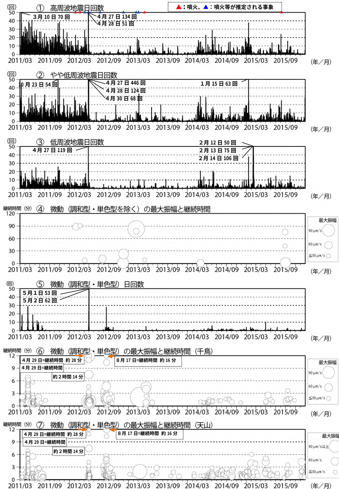
図7 硫黄島 火山活動経過図（2011年3月8日～2015年12月31日）
