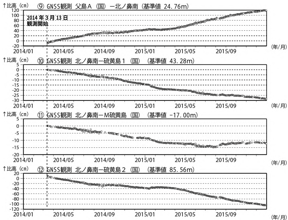
図9 硫黄島 GNSS 観測結果（2014 年 1 月～2015 年 12 月）（国）：国土地理院
