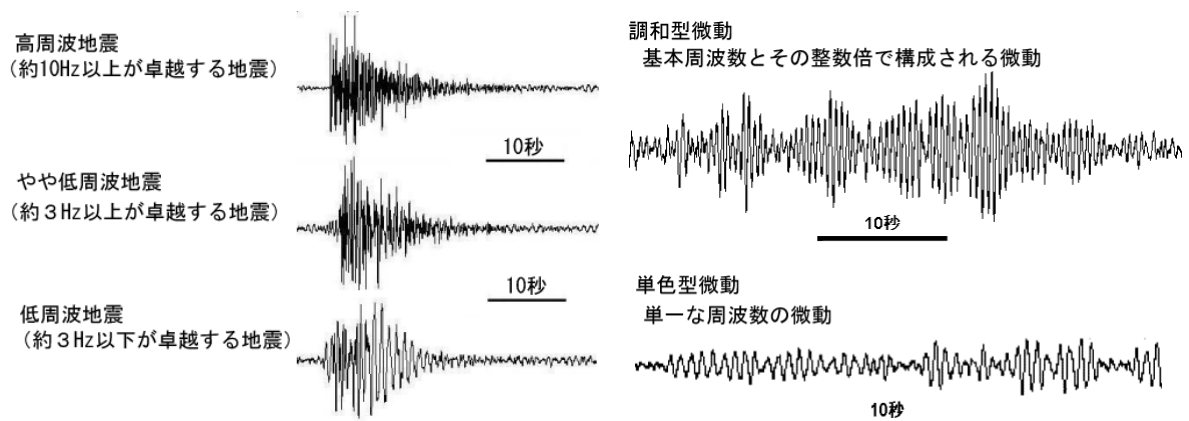
図 6 硫黄島でみられる主な火山性地震、微動（調和型、単色型）の特徴と波形例
