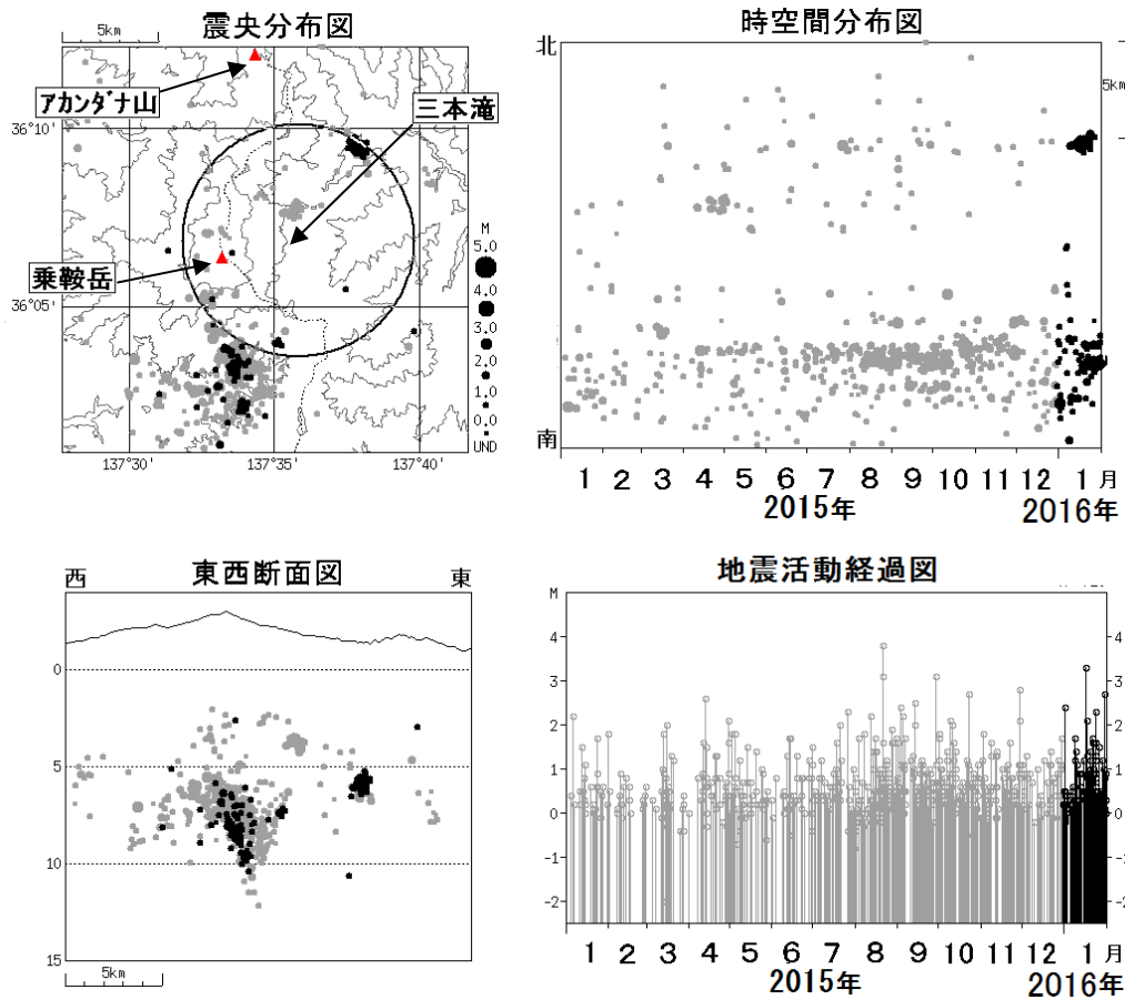
図3 乗鞍岳 広域地震観測網による山体・周辺の地震活動(2015 年 1 月 1 日～2016 年 1 月 31 日)
