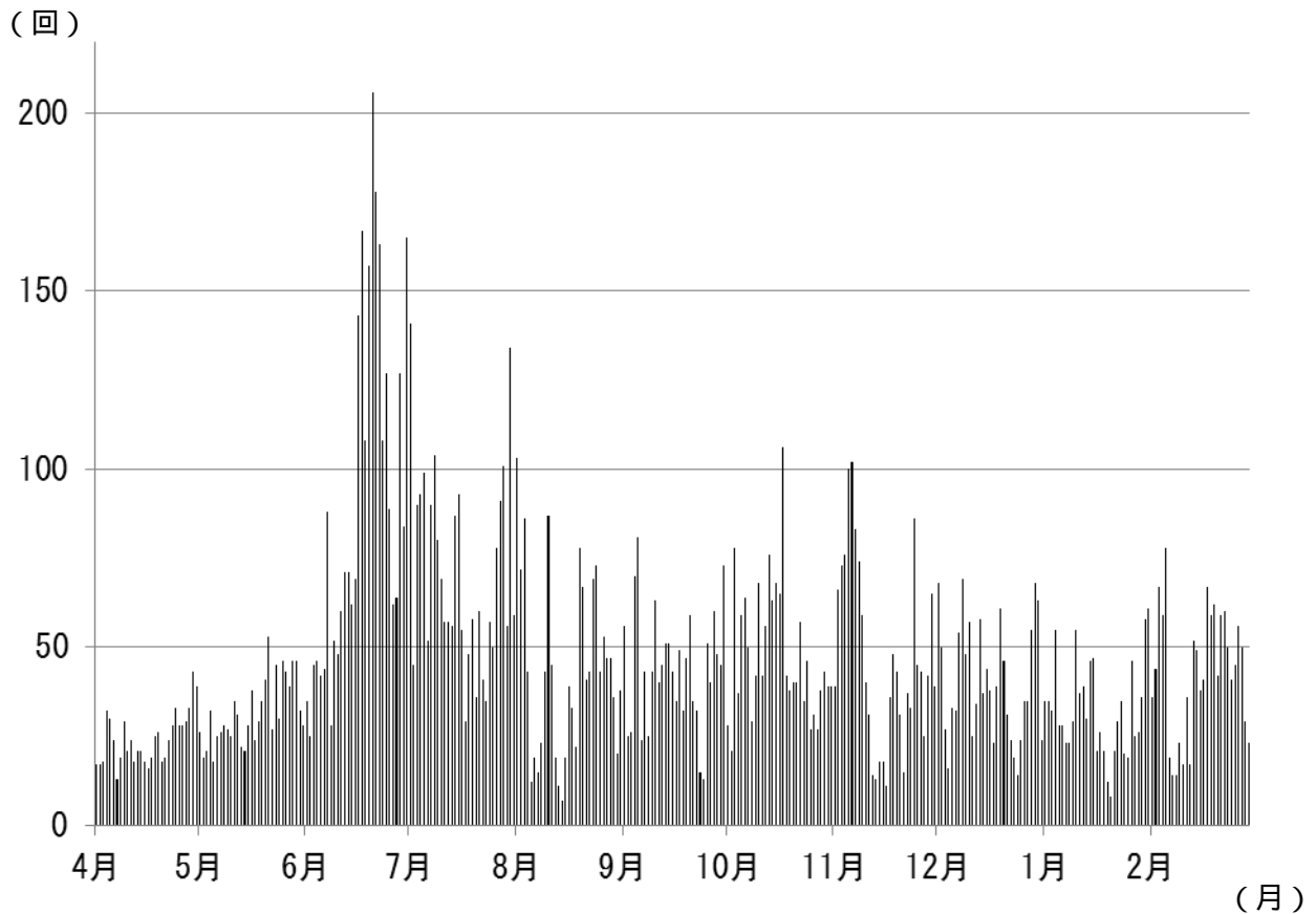
図5 浅間山 火山性地震の日別回数（2015 年 4 月 1 日～2016 年 2 月 29 日）
