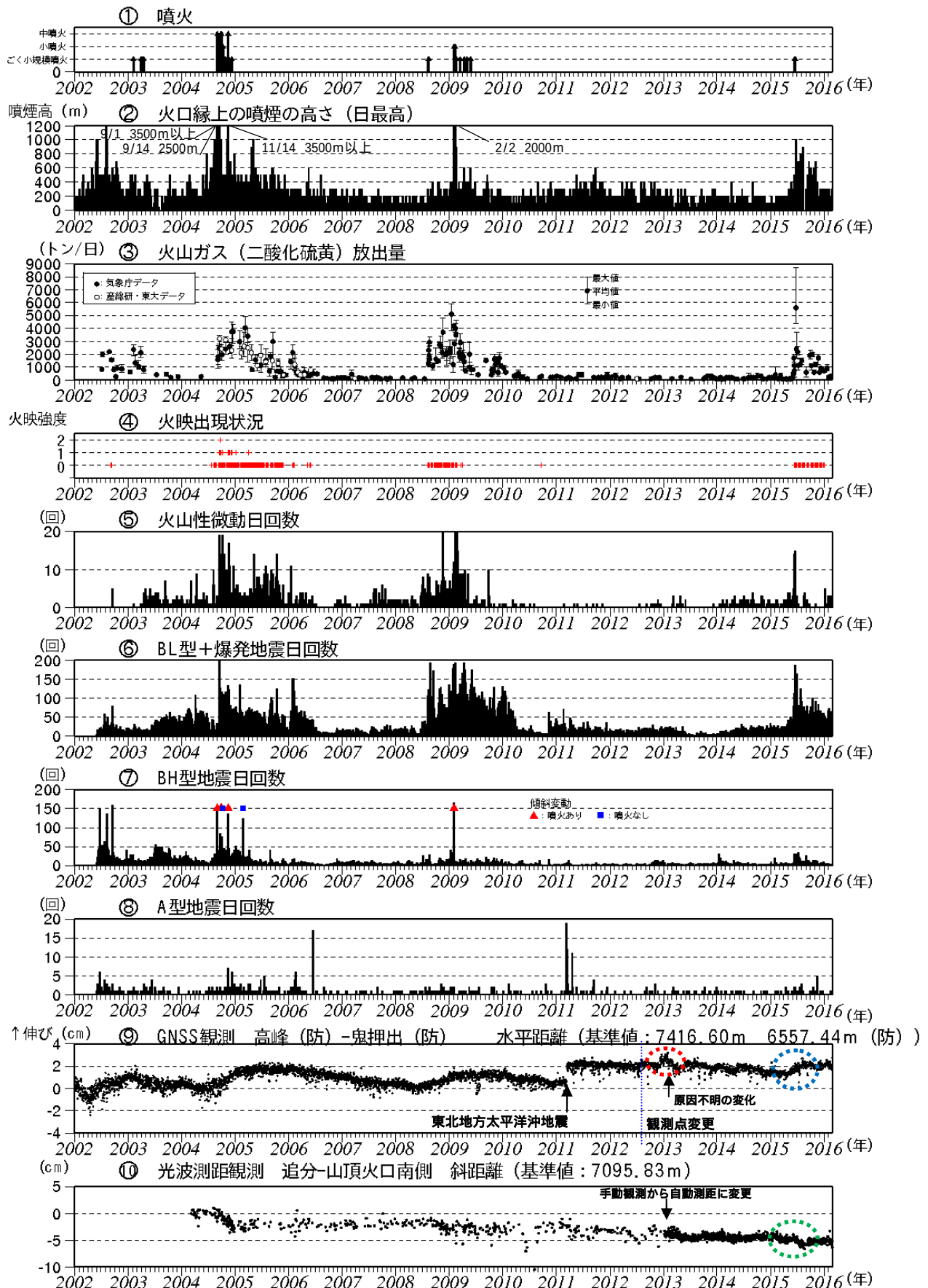
図2 浅間山 火山活動経過図 (2002年1月1日～2016年2月29日)
