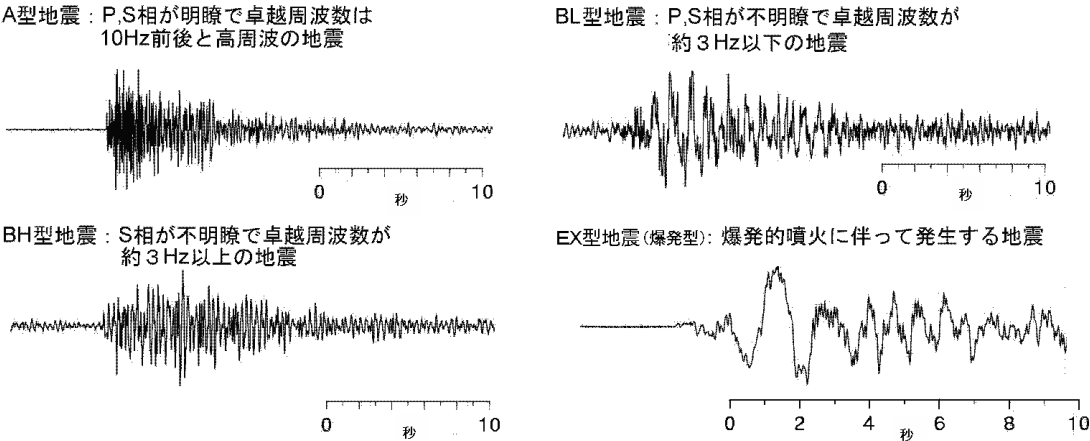
図 10 浅間山で見られる火山性地震の特徴と波形例
