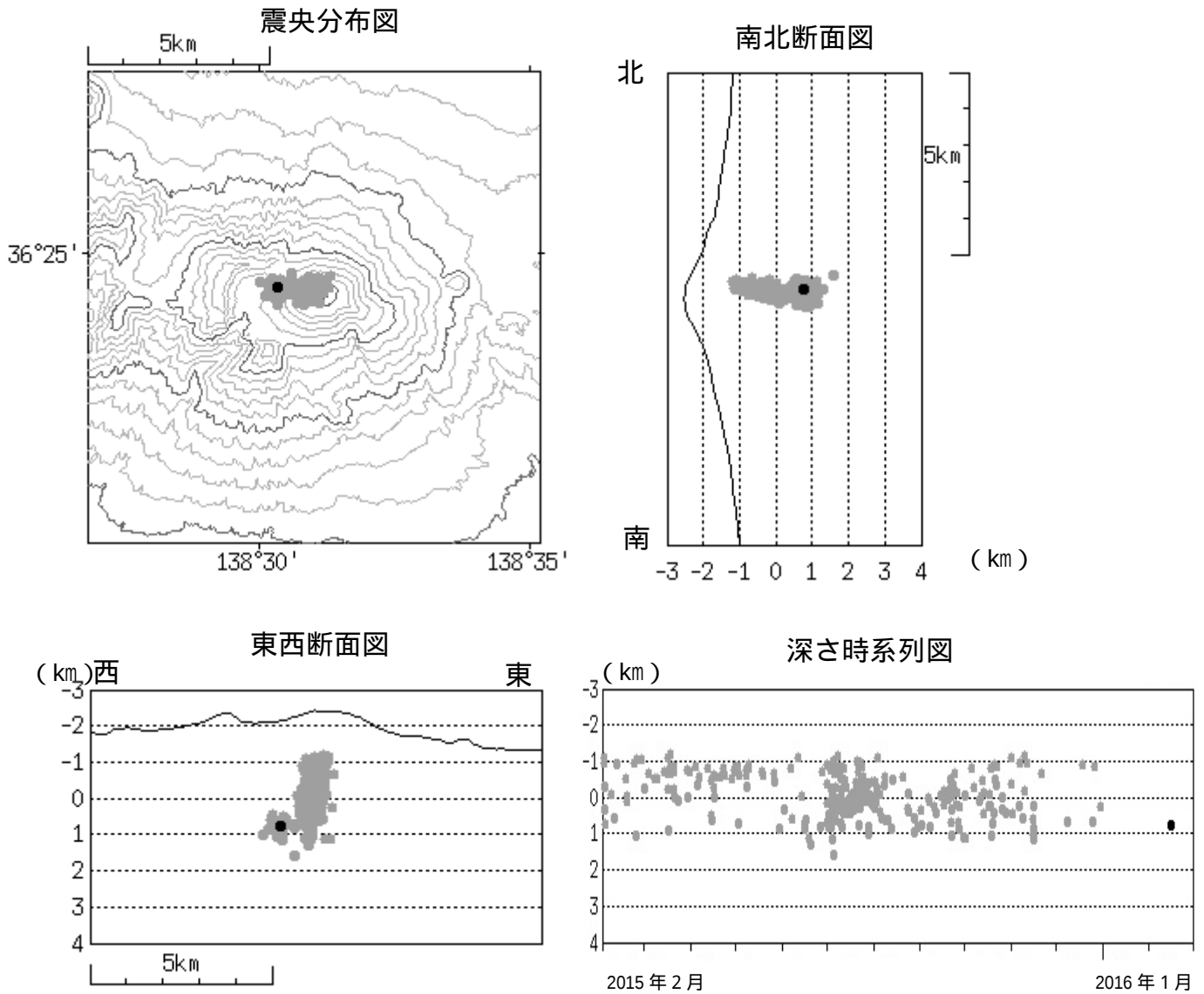
図 4 浅間山 震源分布図（2015 年 2 月 1 日～2016 年 2 月 29 日）
