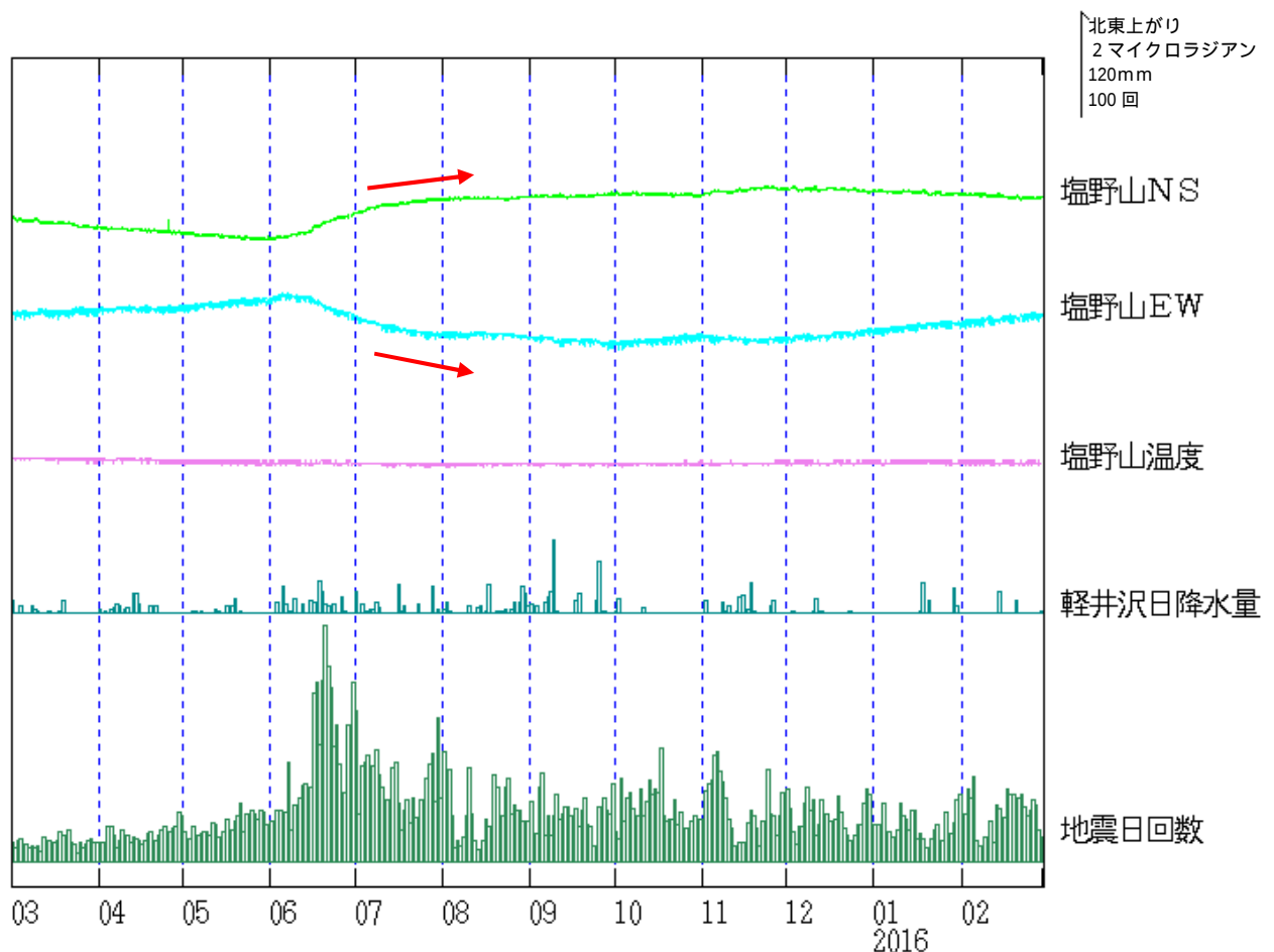
図 9 浅間山 塩野山観測点における傾斜データ（2015 年 3 月 1 日～2016 年 2 月 29 日）
