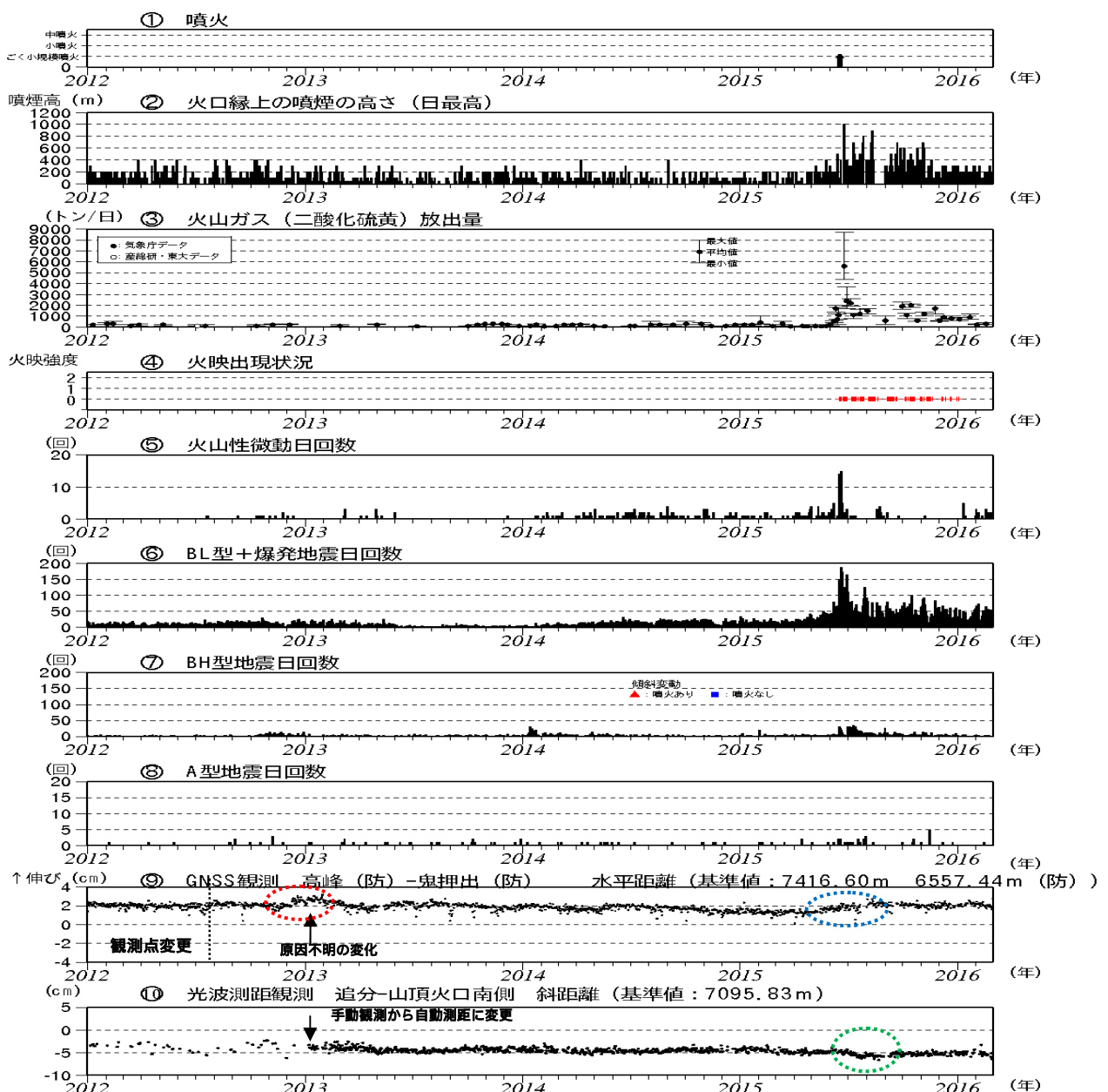
図 3 浅間山 最近の火山活動経過図（2012 年 1 月 1 日 ~ 2016 年 2 月 29 日）
