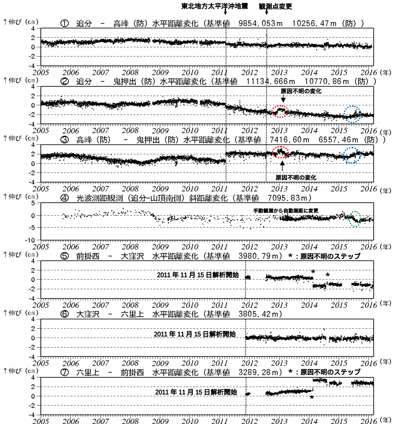
図 7 浅間山 GNSS 連続観測及び光波測距観測の結果(2005 年 1 月 1 日～2016 年 2 月 29 日)
