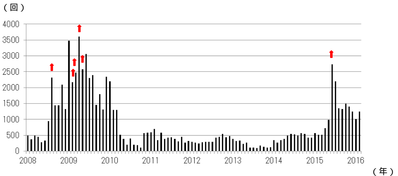
図6 浅間山 火山性地震の月別回数（2008 年 1 月～2016 年 2 月）
