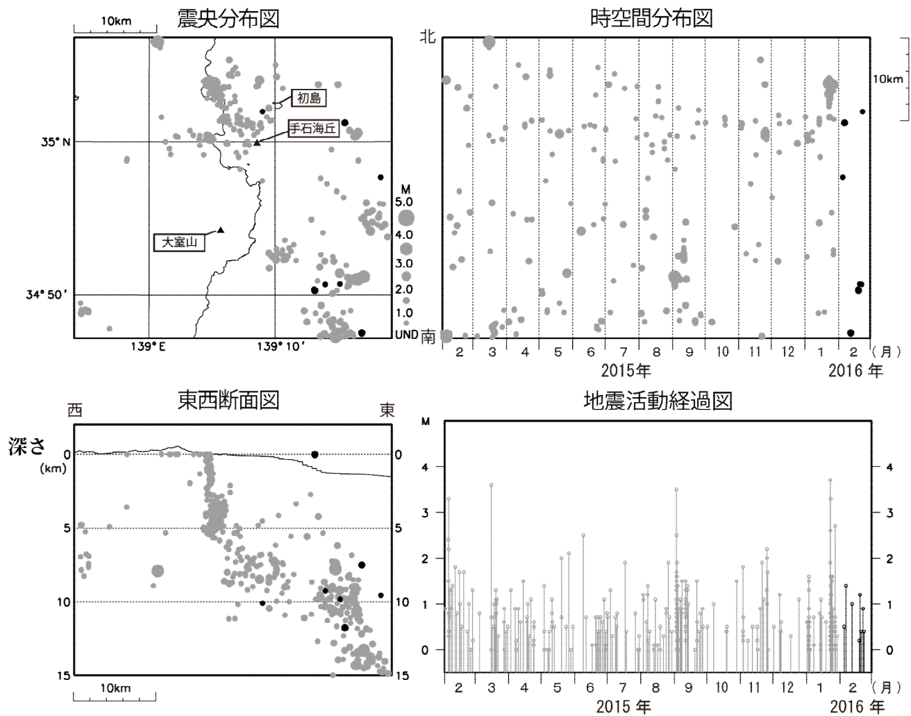
●：2015年2月1日～2016年1月31日 ●：2016年2月1日～2月29日 図2 伊豆東部火山群 広域地震観測網による震源分布図（2015年2月1日～2016年2月29日） ・ M（マグニチュード）は地震の規模を表します。 ・ 図中の震源要素は一部暫定値が含まれており、後日変更することがあります。
