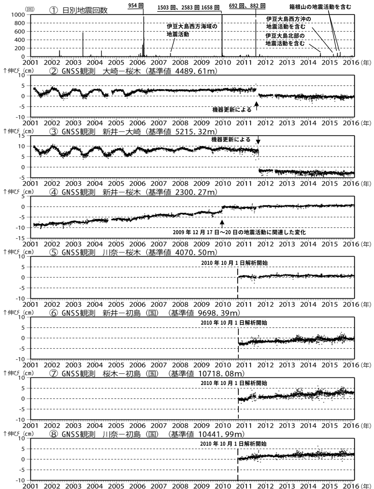
図3 伊豆東部火山群 火山活動経過図（2001年1月1日～2016年2月29日）
