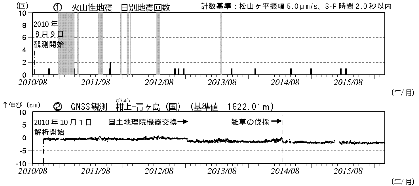
図 2 青ヶ島 火山活動経過図 (2010 年 8 月 9 日 ~ 2016 年 2 月 29 日) 青ヶ島周辺の日別地震回数 グラフの灰色部分は機器障害による欠測。 GNSS 連続観測による基線長変化 (国): 国土地理院 は図 3 の GNSS 基線 に対応。グラフの空白部分は欠測。 ・2014 年 7 月 15 日に実施した雑草の伐採の影響により、ステップ状の変化がみられます。
