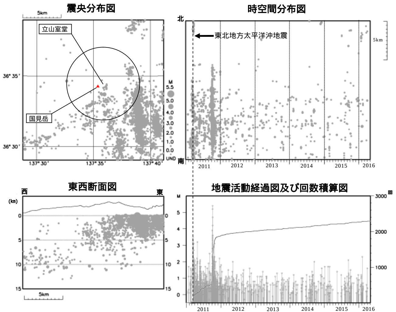
図 2 弥陀ヶ原 広域地震観測網による山体・周辺の地震活動（2011 年 1 月 1 日～2016 年 4 月 30 日）
