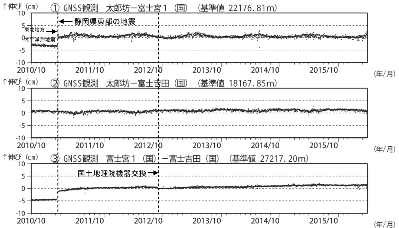
図 4 富士山 GNSS 連続観測による基線長変化（2010 年 10 月 1 日～2016 年 6 月 30 日） （国）：国土地理院
