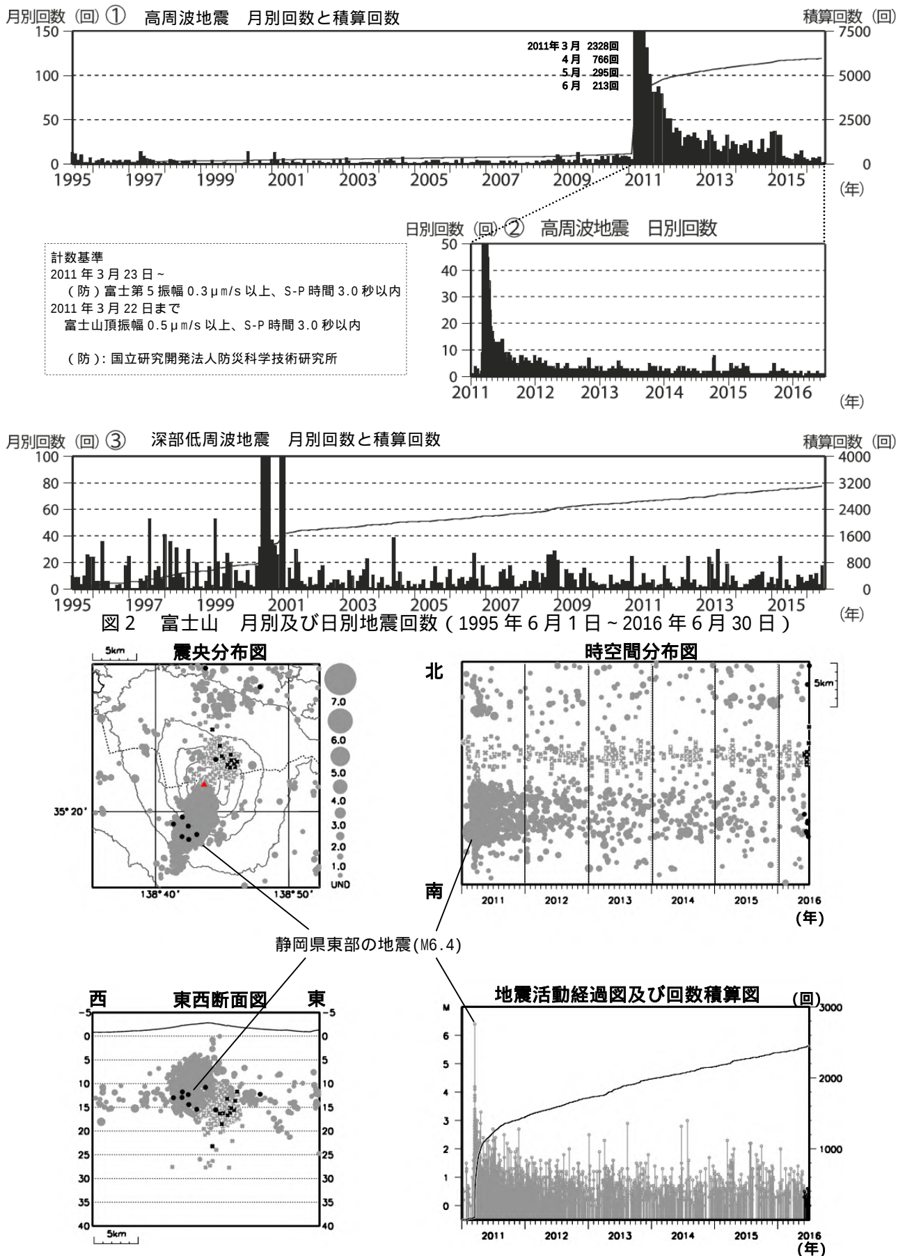
図 3 富士山 広域地震観測網による山体・周辺の地震活動 (2011 年 1 月 1 日～2016 年 6 月 30 日)
