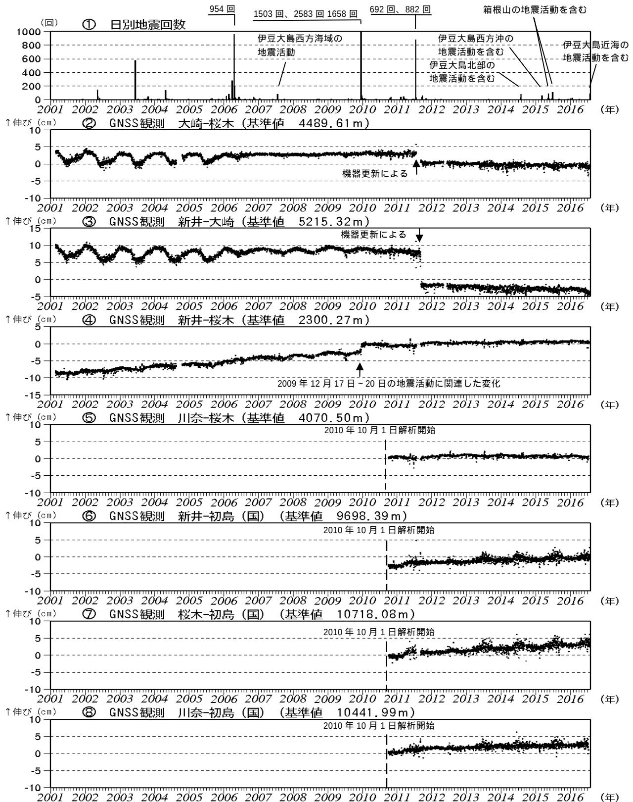
図3 伊豆東部火山群 火山活動経過図(2001年1月1日~2016年7月31日)
