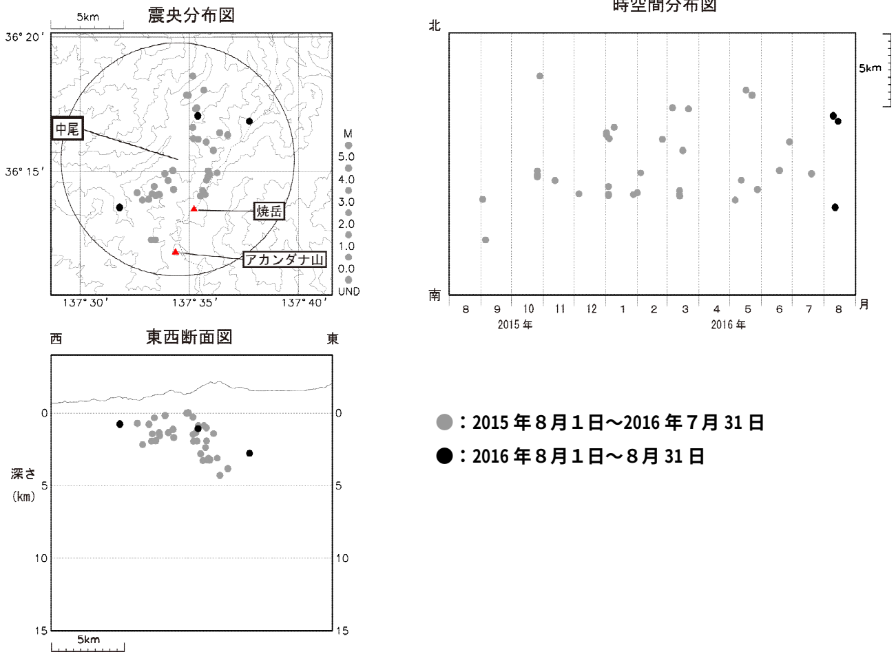
図 3 焼岳 震源分布図（2015 年 8 月 1 日～2016 年 8 月 31 日）
