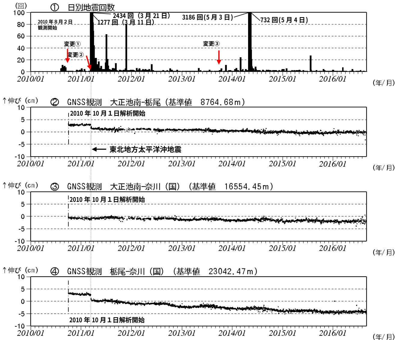
図 2 焼岳 火山活動経過図（2010年8月2日～2016年8月31日）
