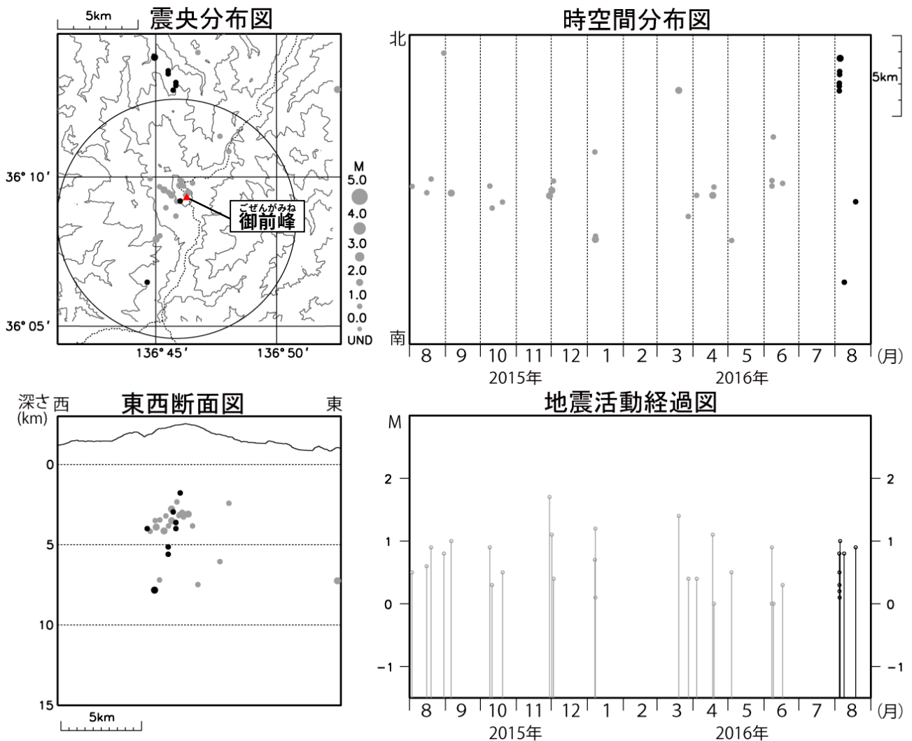
図4 白山 広域地震観測網による山体・周辺の地震活動（2015 年 8 月 1 日～2016 年 8 月 31 日）
