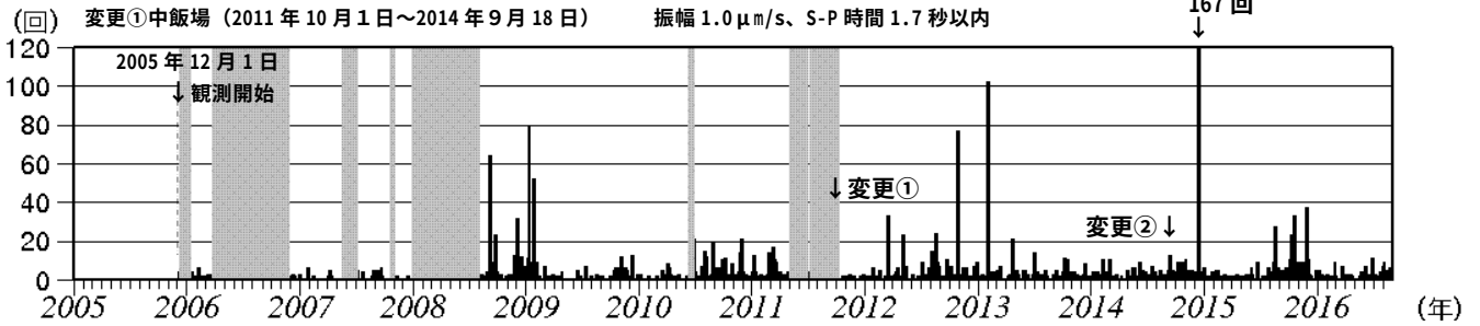
図3 白山 日別地震回数（2005 年 12 月 1 日～2016 年 8 月 31 日）
