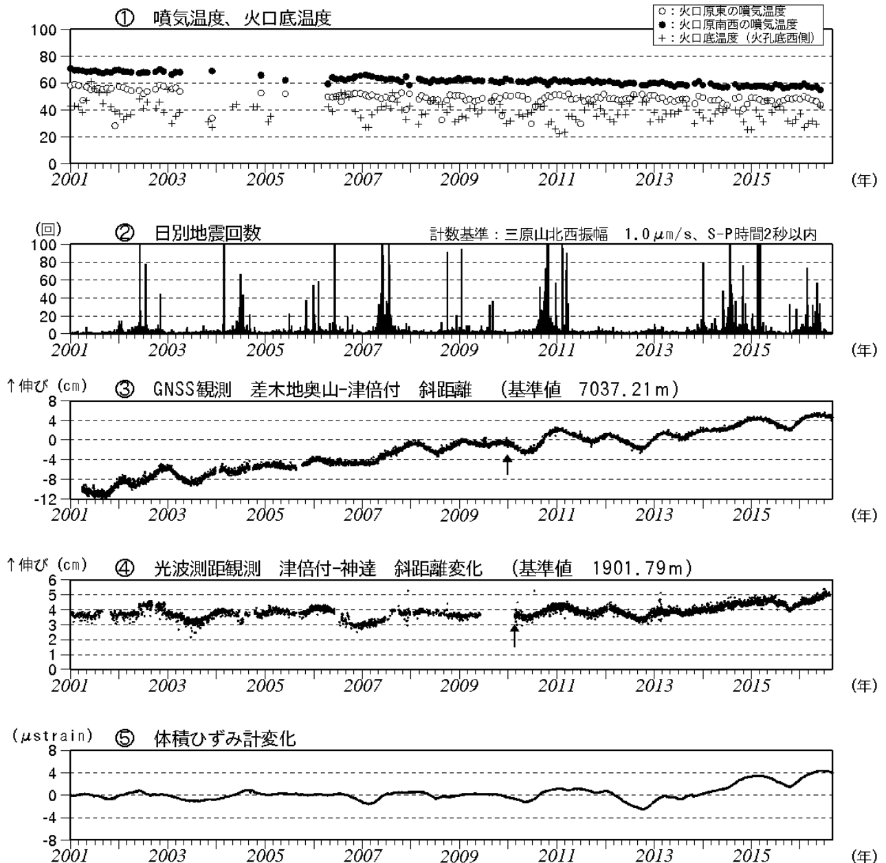
図2 伊豆大島 最近の火山活動経過図（2001年1月～2016年8月31日）
