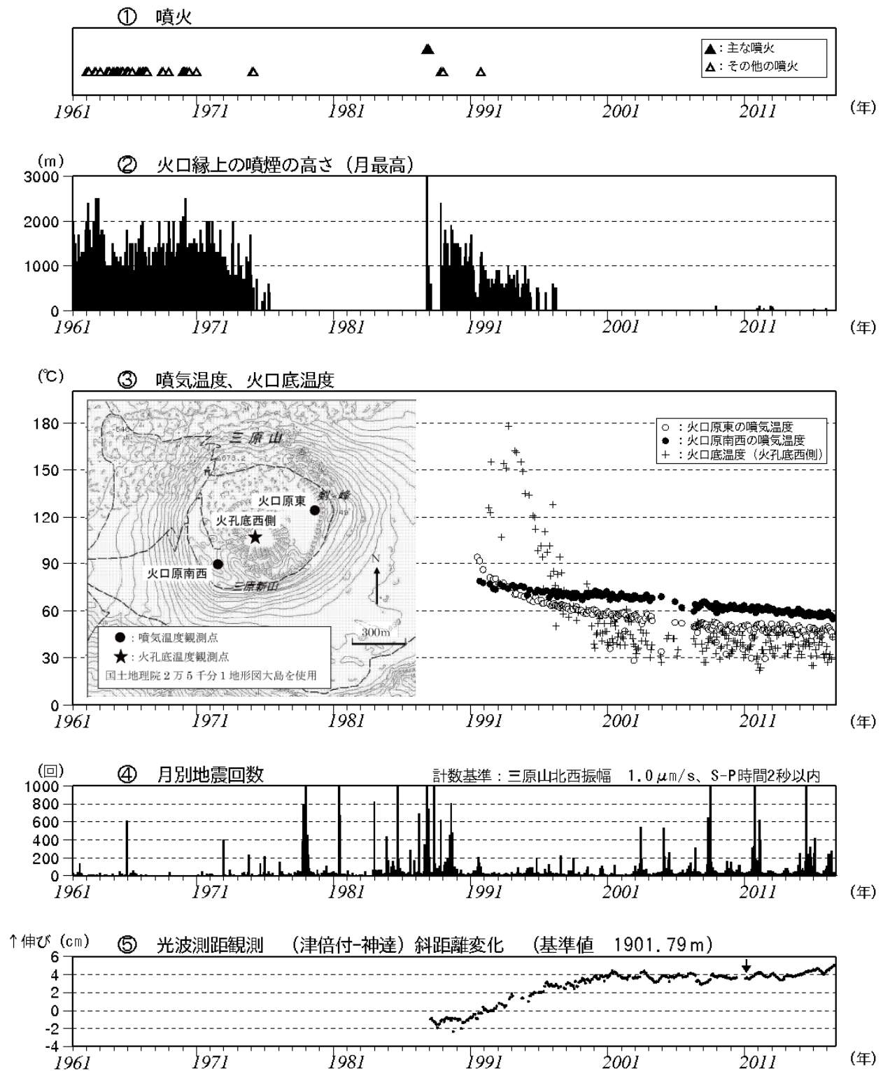
図 1 伊豆大島 長期間の火山活動経過図（1961 年 1 月～2016 年 8 月 31 日）
