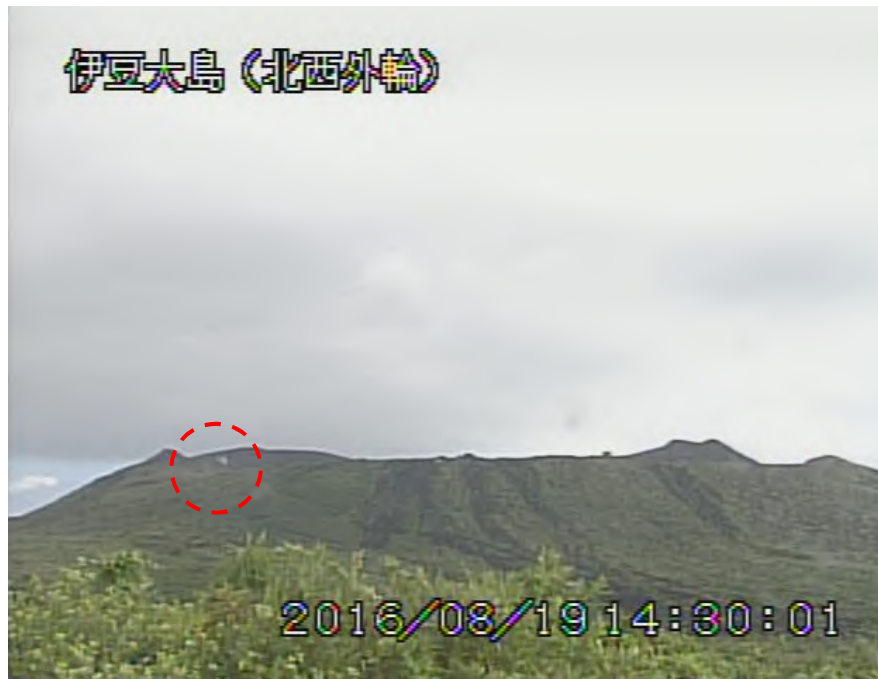
図5 伊豆大島 三原山山頂部の状況 山頂部（8月19日、北西外輪遠望カメラによる） 破線円内：ごく弱い噴気
