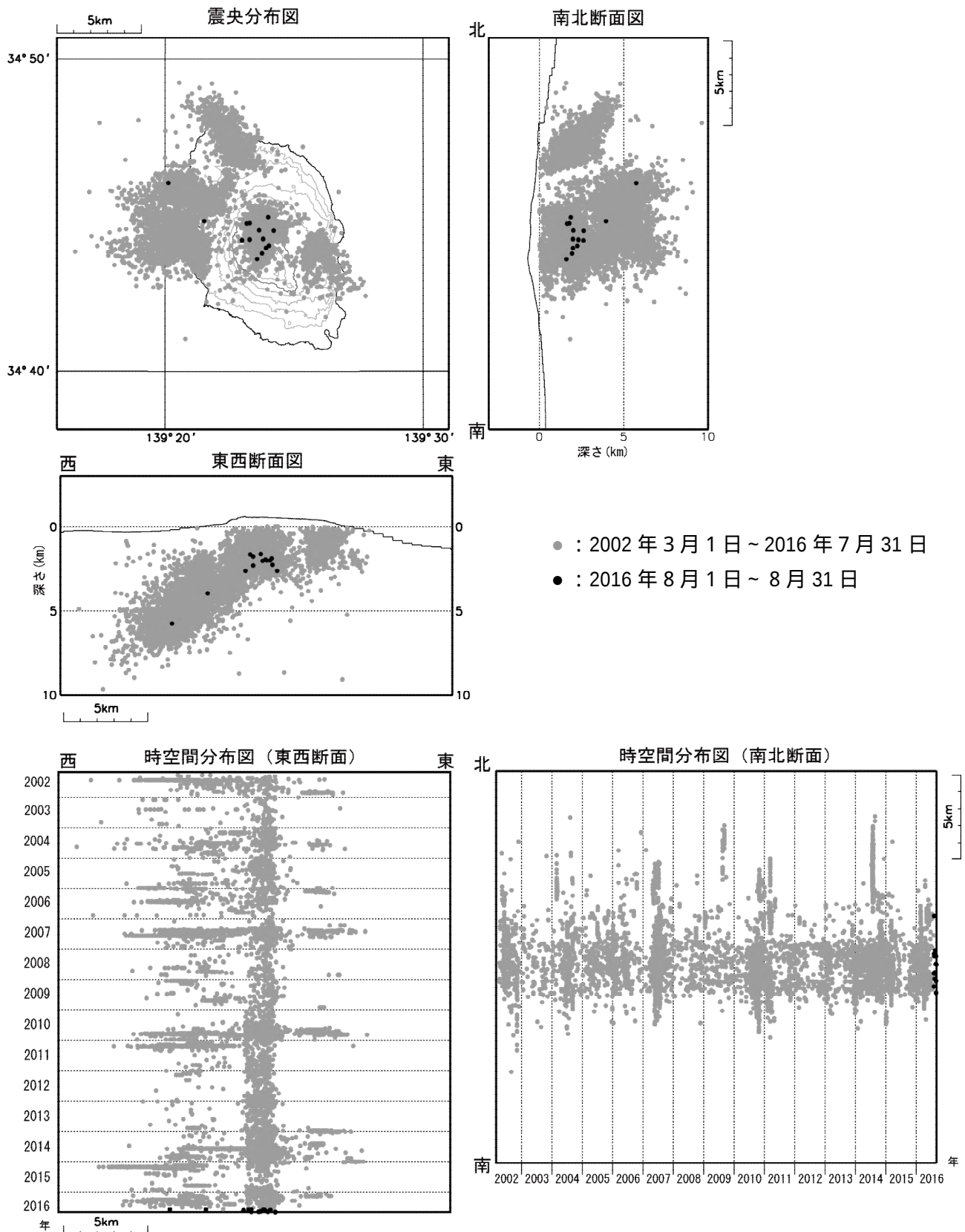
図 4 伊豆大島 震源分布図（2002 年 3 月 1 日～2016 年 8 月 31 日）
