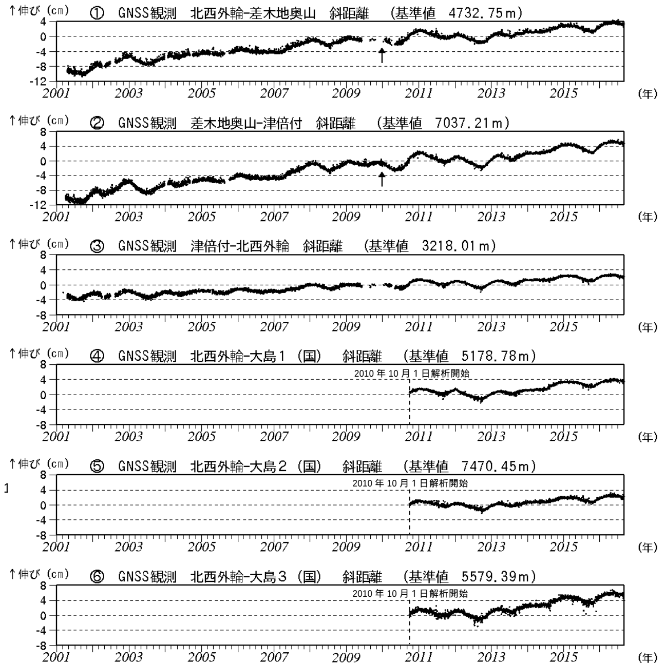
図3 伊豆大島 GNSS連続観測による基線長変化(2001年1月～2016年8月31日)(国): 国土地理院 2010年10月以降のデータについては、電離層の影響を補正する等、解析方法を改良しています。
