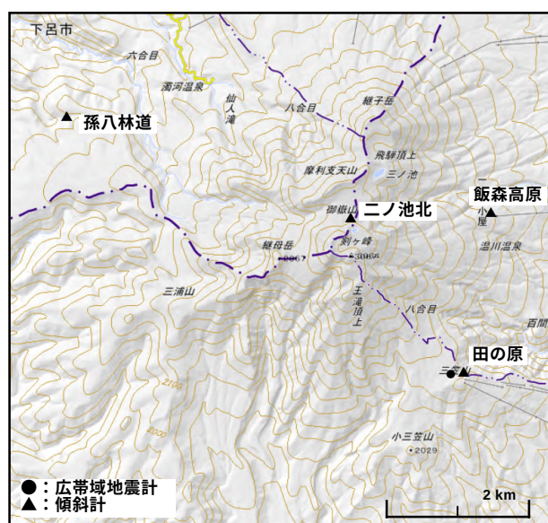
図7 図6中の地震計と傾斜計の観測点配置図
