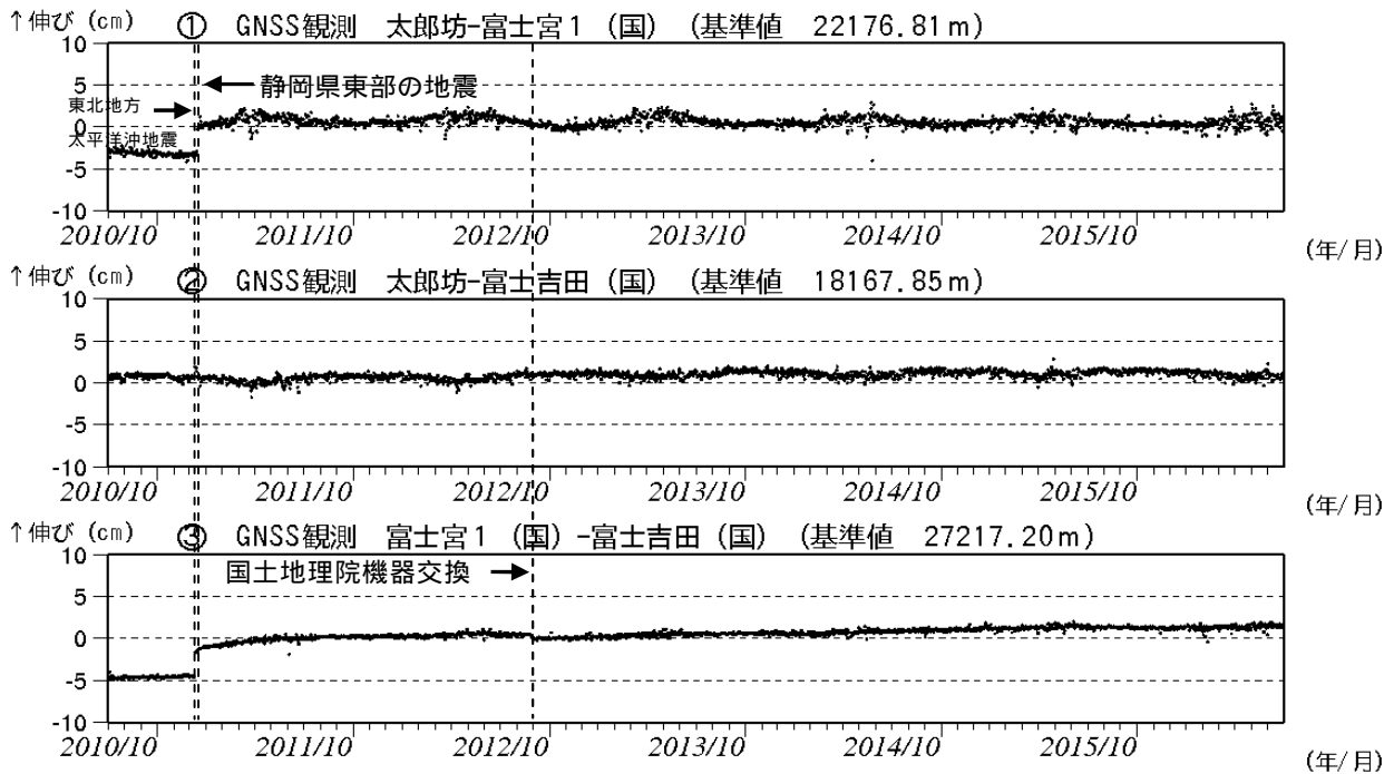
図4 富士山 GNSS 連続観測による基線長変化（2010 年 10 月 1 日～2016 年 9 月 30 日）
