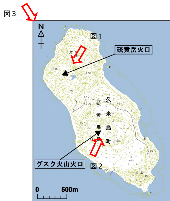
図 4 硫黄島 火口位置図と各図の撮影方向
