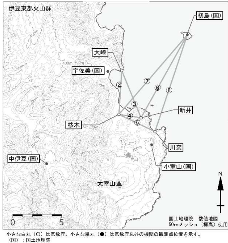
図 4 伊豆東部火山群 GNSS 連続観測点配置図 ・ 図中の GNSS 基線 ~ は図 3 の ~ に対応しています。
