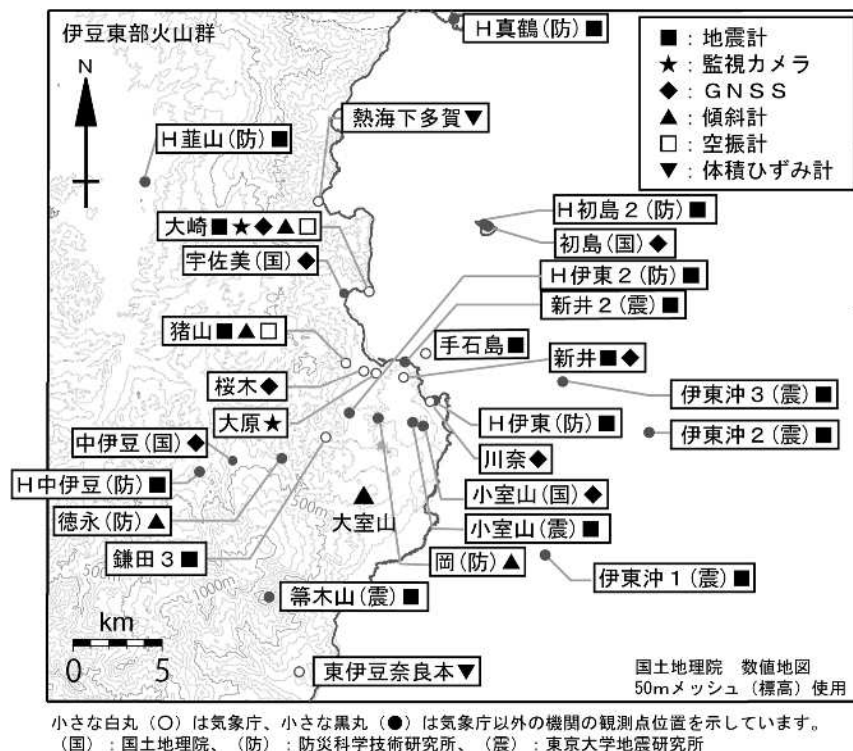
図 5 伊豆東部火山群 観測点配置図 手石島：12 月 1 日運用開始。
