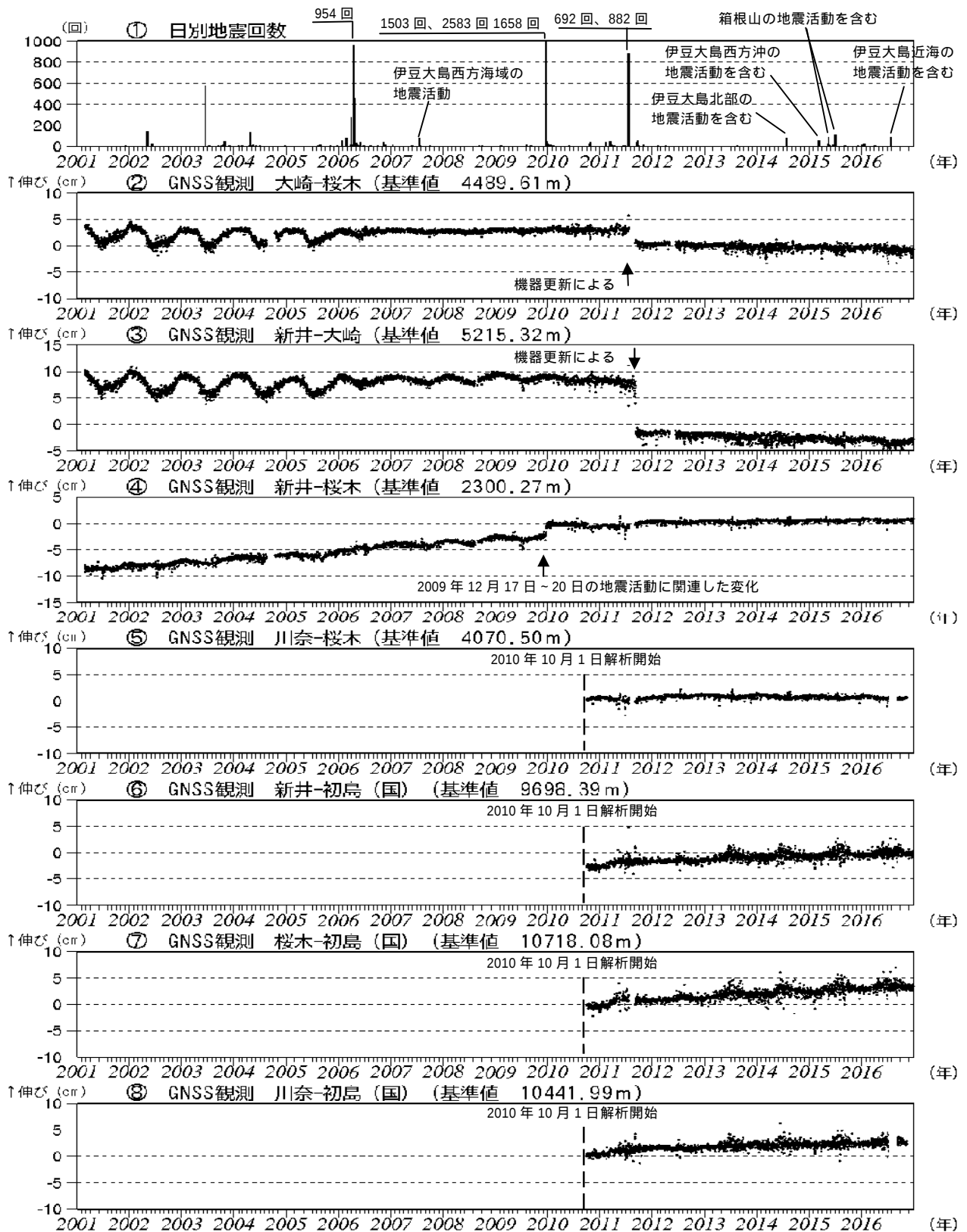
図3 伊豆東部火山群 火山活動経過図（2001年1月1日～2016年12月31日）
