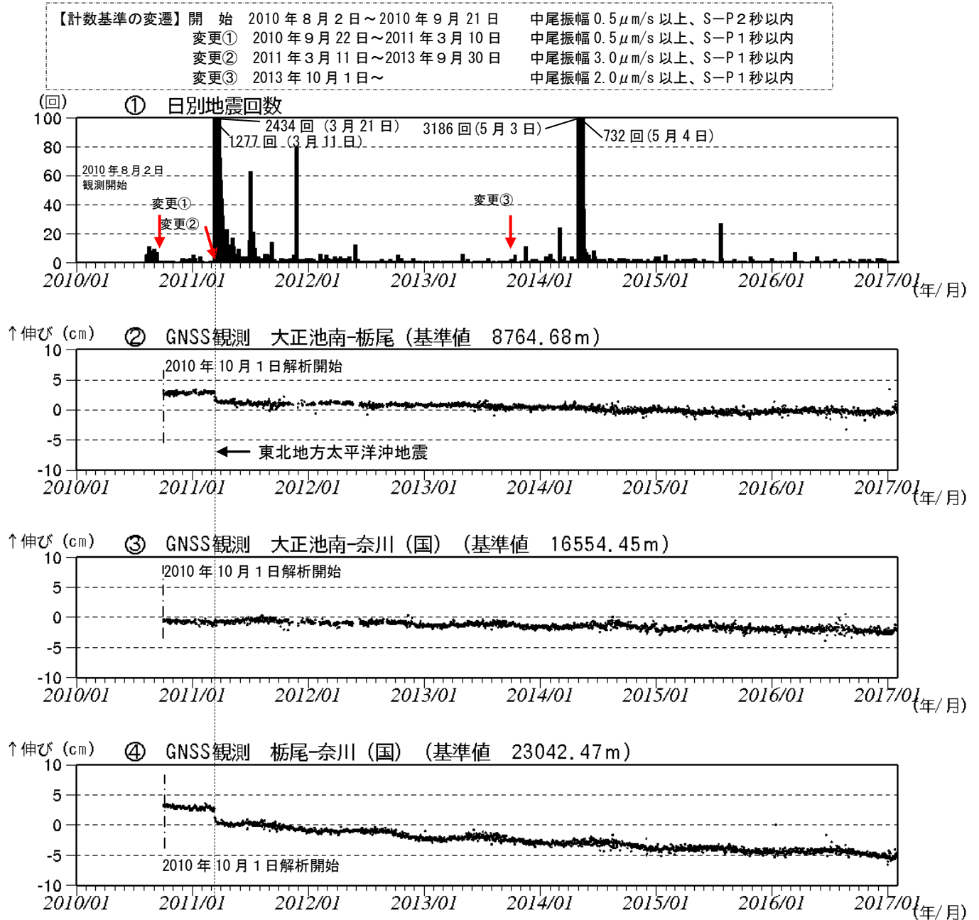
図 2 焼岳 火山活動経過図（2010年 8 月 2 日～2017年 1 月 31 日）
