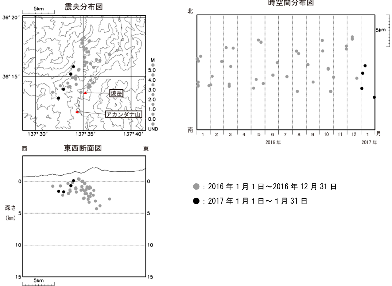
図 3 焼岳 震源分布図（2016 年 1 月 1 日～2017 年 1 月 31 日）
