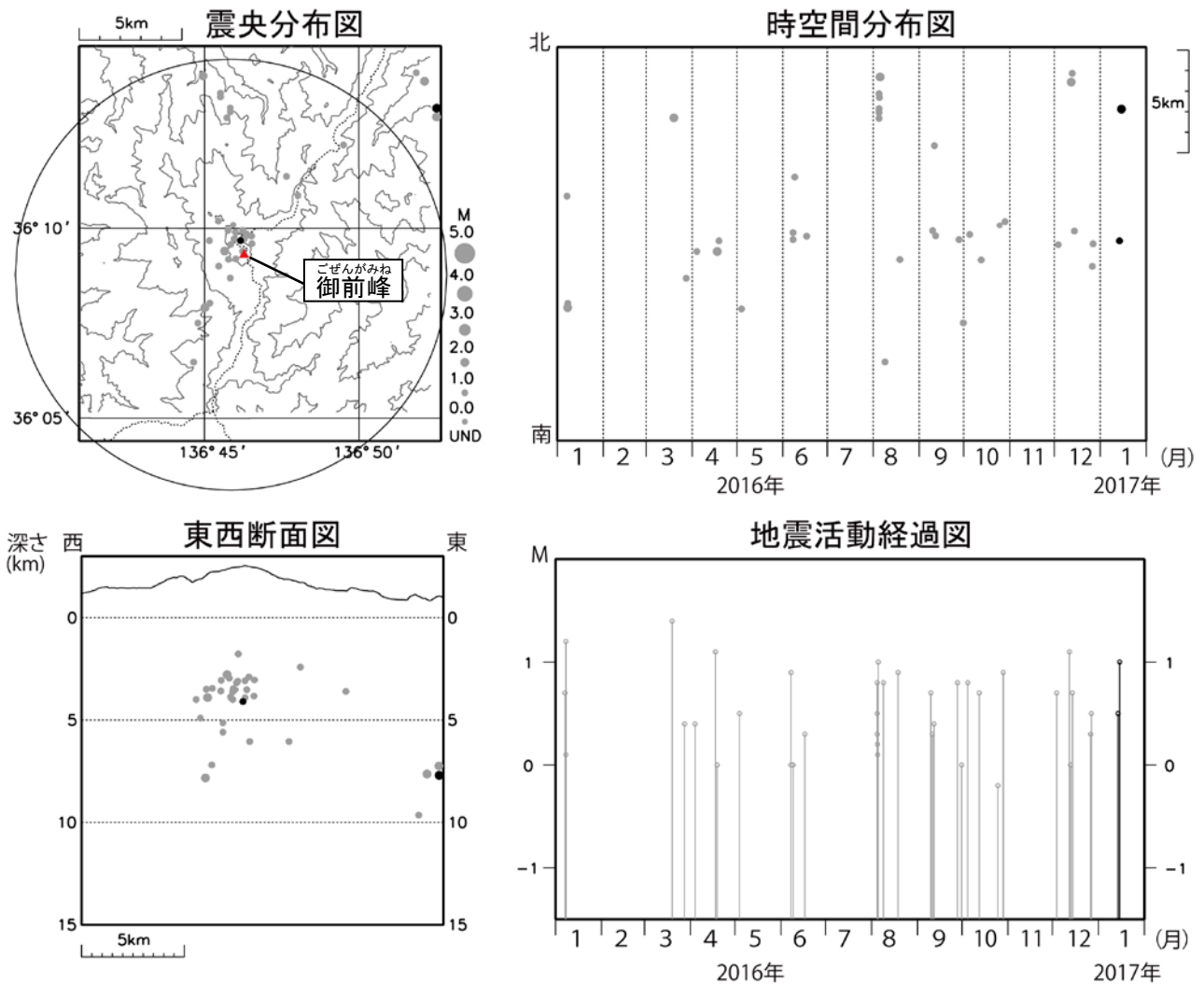
図 4 白山 広域地震観測網による山体・周辺の地震活動（2016 年 1 月 1 日～2017 年 1 月 31 日）
