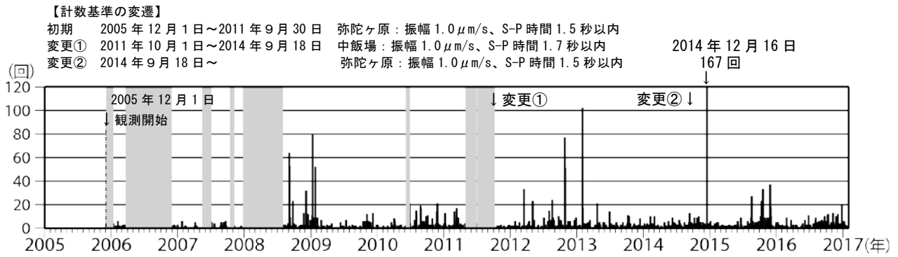
図 3 白山 日別地震回数（2005 年 12 月 1 日～2017 年 1 月 31 日） ・図の灰色部分は機器障害による欠測期間
