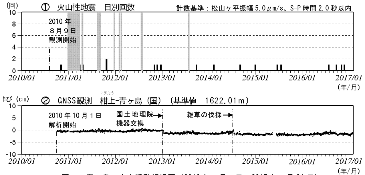
図2 青ヶ島 火山活動経過図（2010年8月9日～2017年1月31日）
