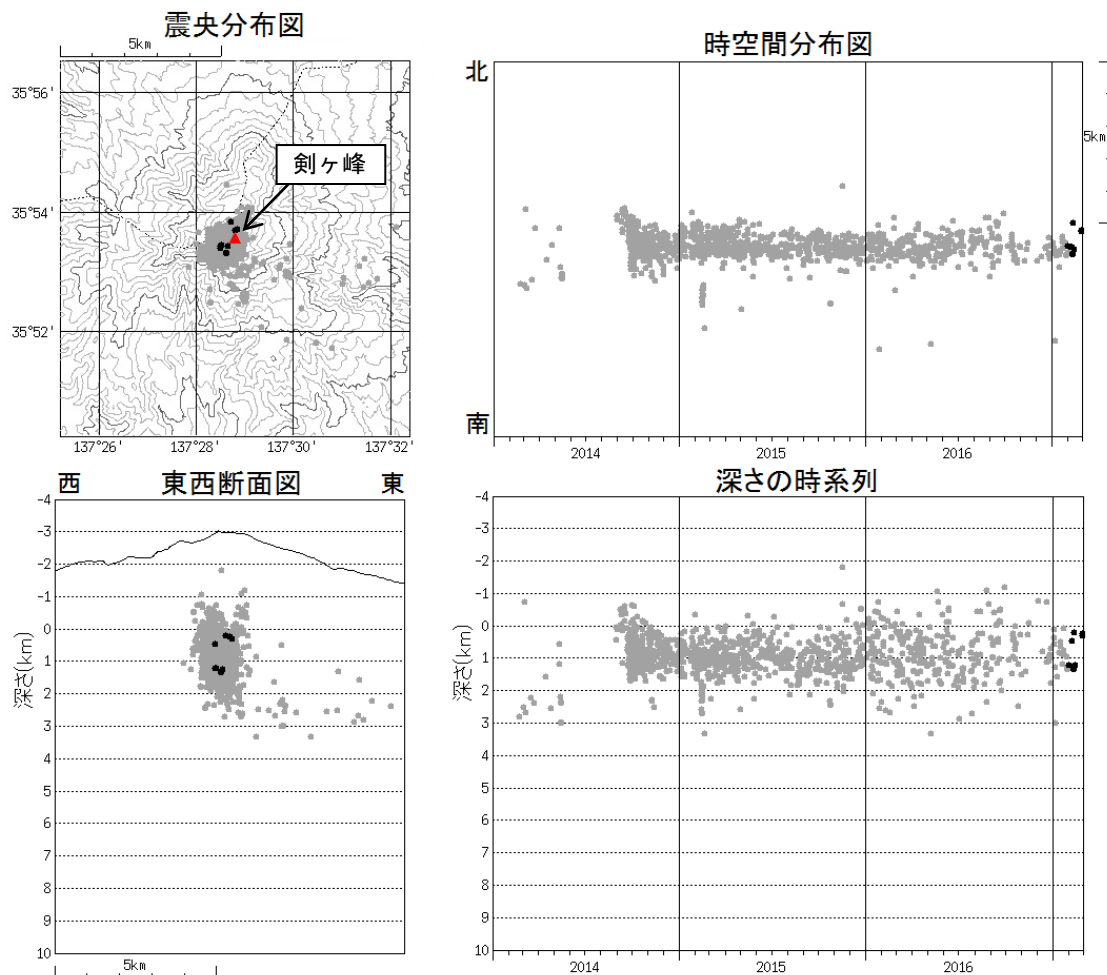
図 2 御嶽山 震源分布図（2014 年 1 月 1 日～2017 年 2 月 28 日）
