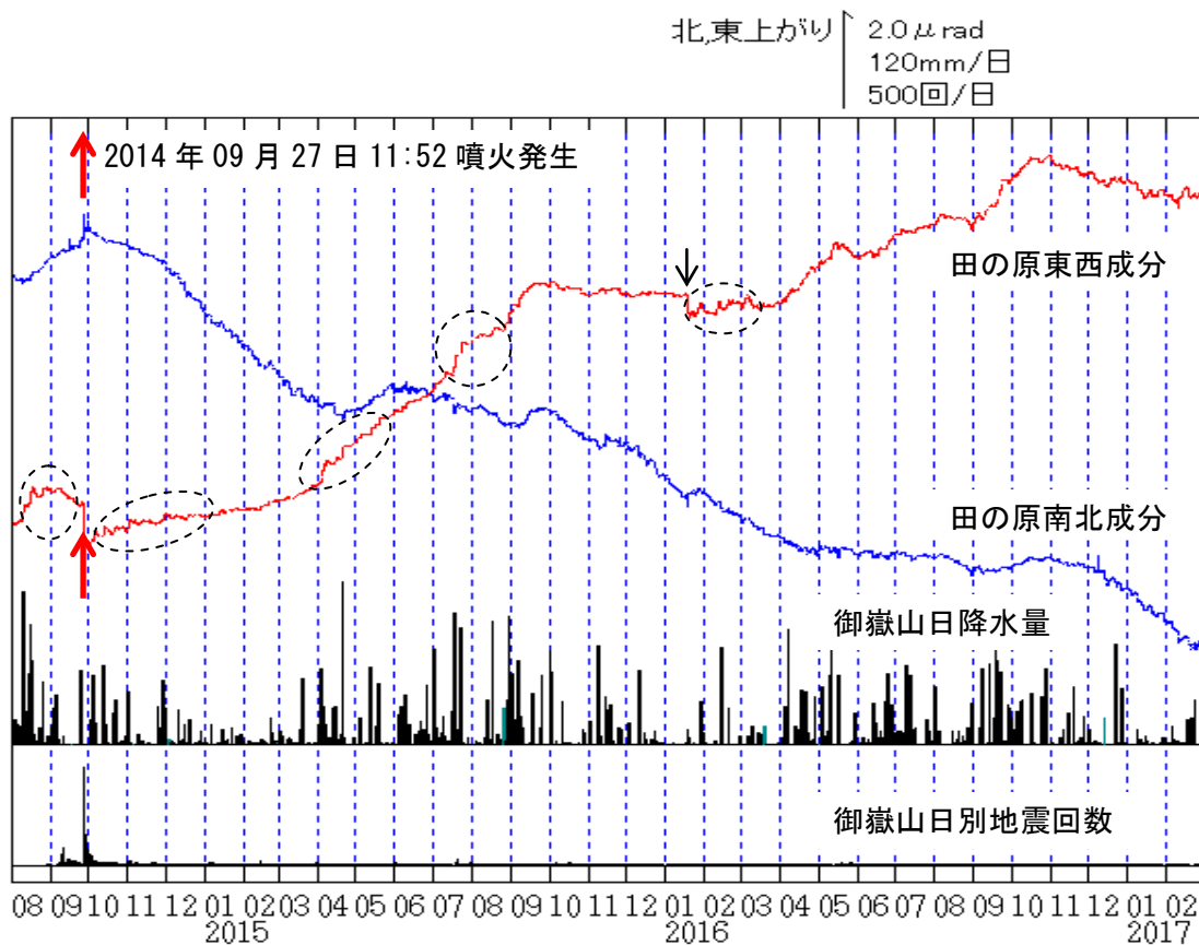
図 6 御嶽山 田の原観測点（剣ヶ峰山頂の南東約 3 km）の傾斜変動 （2014 年 8 月 1 日～2017 年 2 月 28 日）
