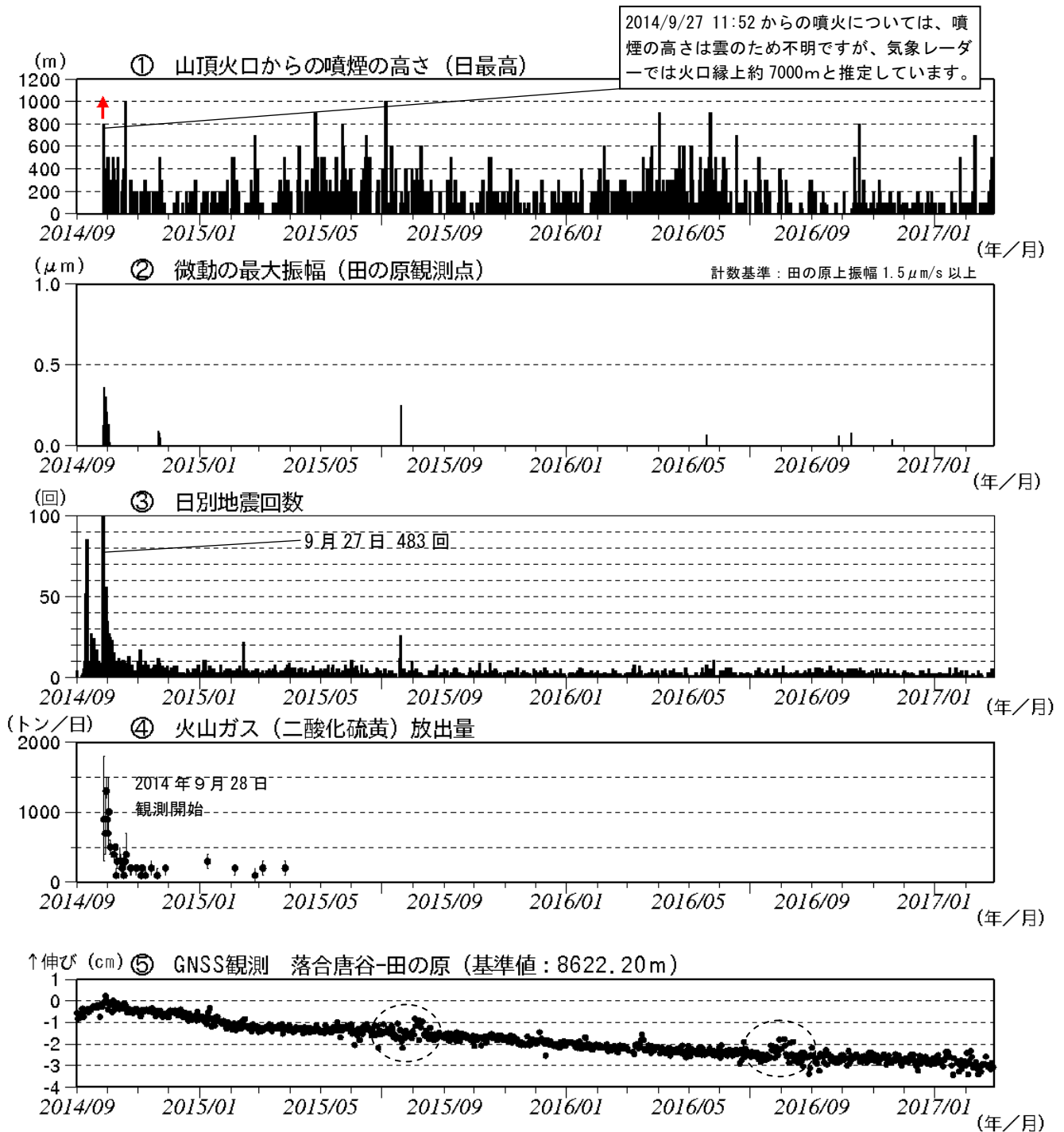
図3 御嶽山 最近の火山活動経過図（2014年9月1日～2017年2月28日）
