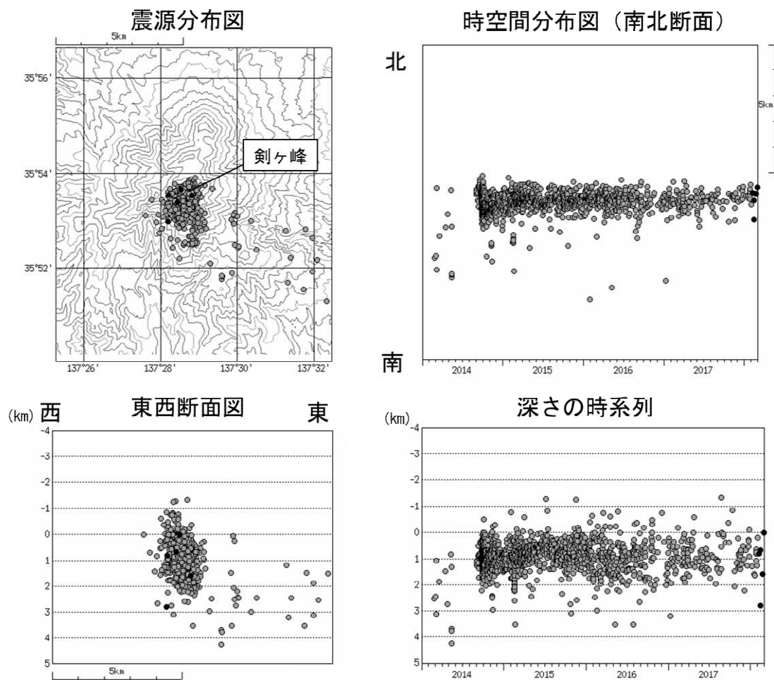
図 2 御嶽山 震源分布図（2014 年 1 月 1 日～2018 年 2 月 28 日）
