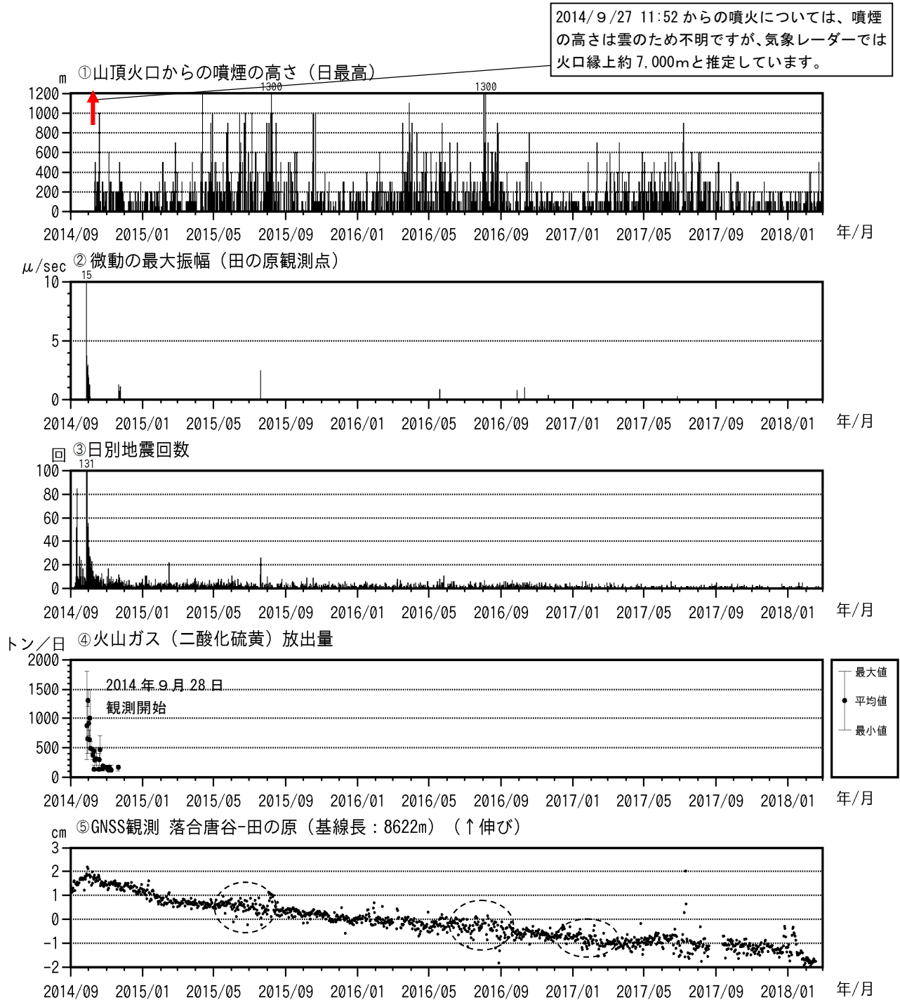
図3 御嶽山 最近の火山活動経過図（2014年9月1日～2018年2月28日）
