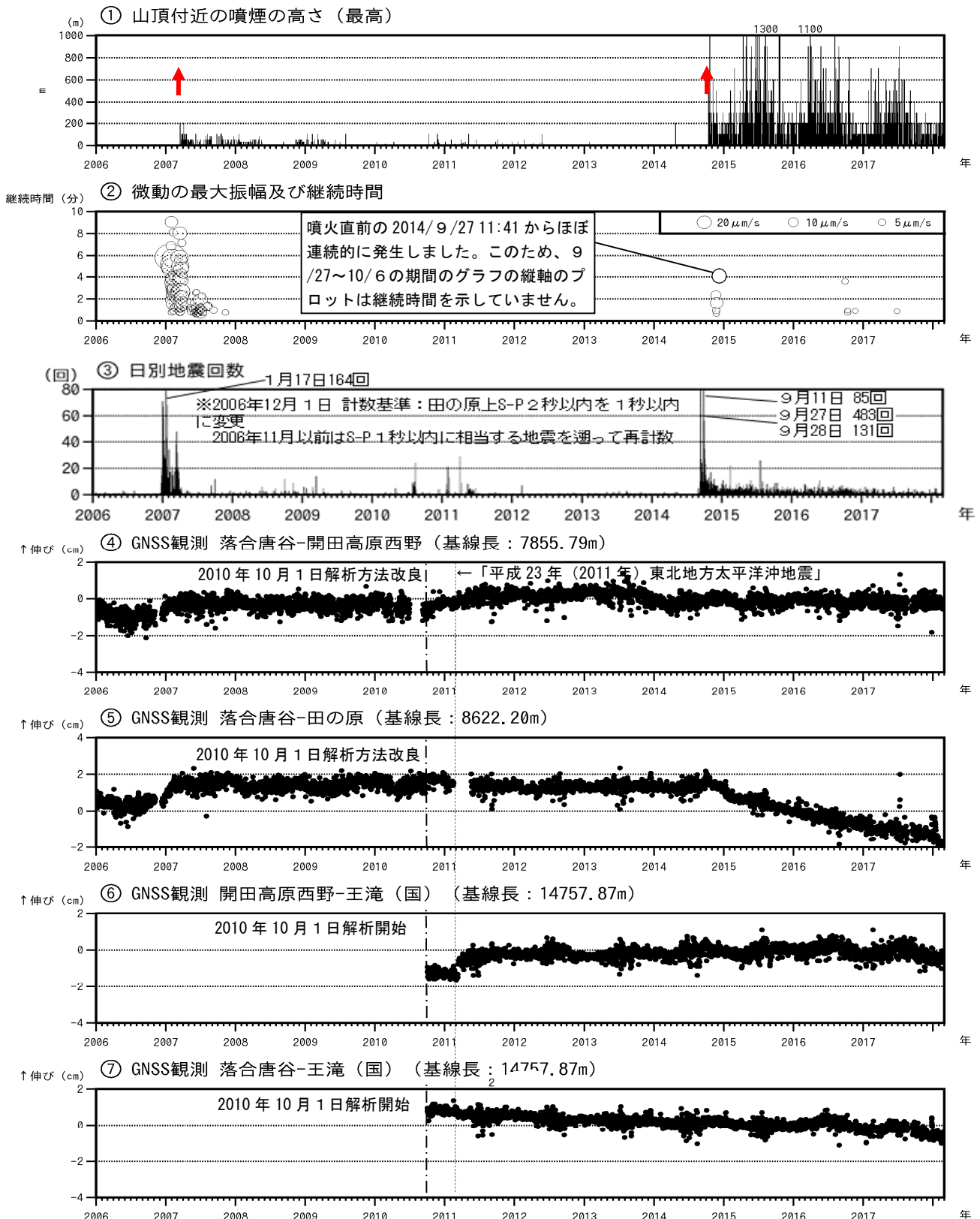
図4 御嶽山 長期間の火山活動経過図（2006年1月1日～2018年2月28日）
