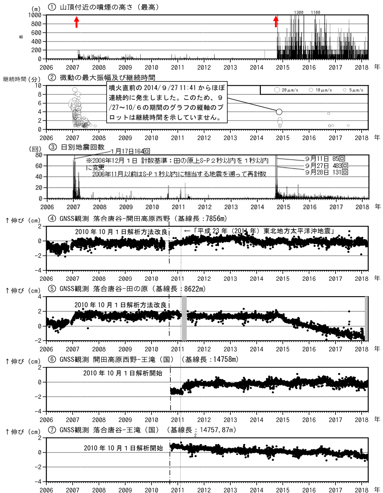
図 4 御嶽山 長期間の火山活動経過図（2006 年 1 月 1 日～2018 年 3 月 31 日）
