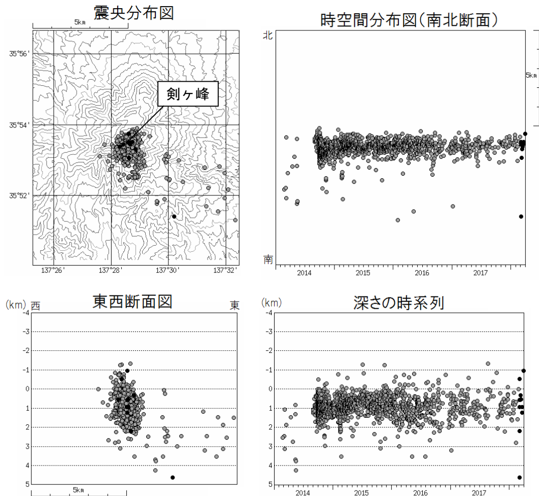
図 2 御嶽山 震源分布図（2014 年 1 月 1 日～2018 年 3 月 31 日）
