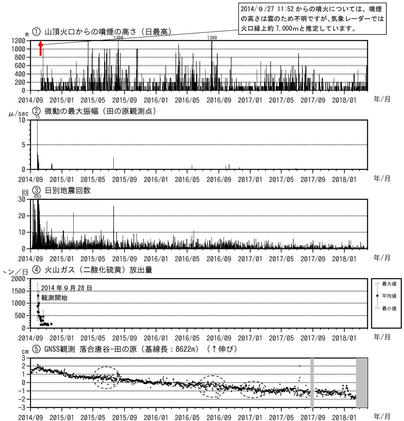
図3 御嶽山 最近の火山活動経過図（2014年9月1日～2018年3月31日）
