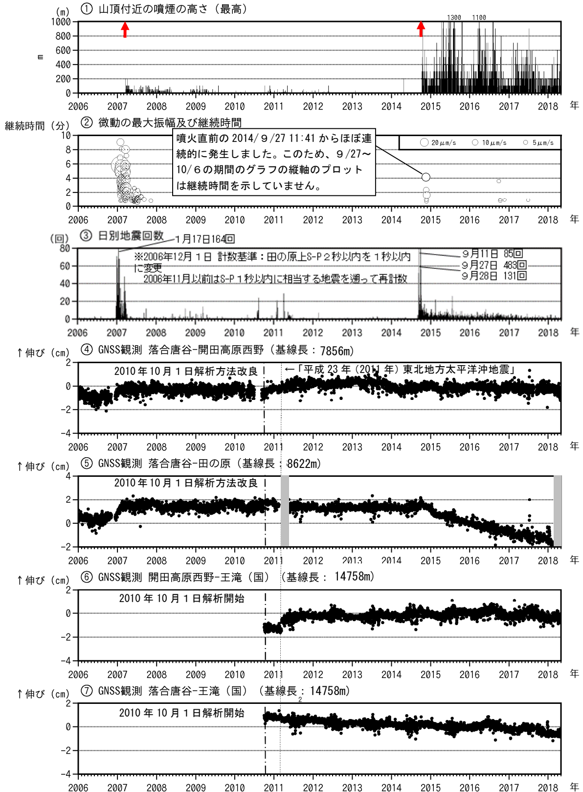
図4 御嶽山 長期間の火山活動経過図（2006年1月1日～2018年4月30日）
