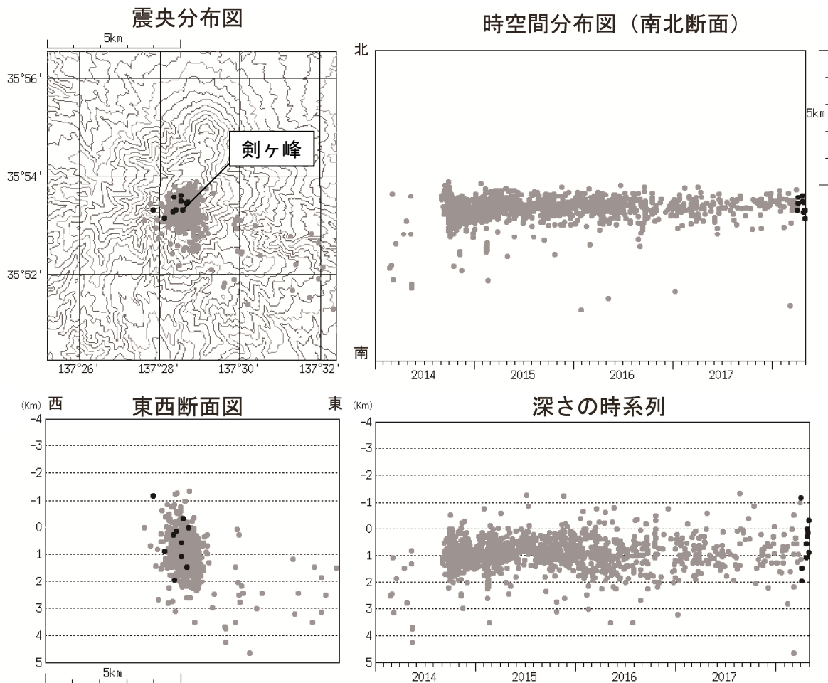
図 2 御嶽山 震源分布図（2014 年 1 月 1 日～2018 年 4 月 30 日）
